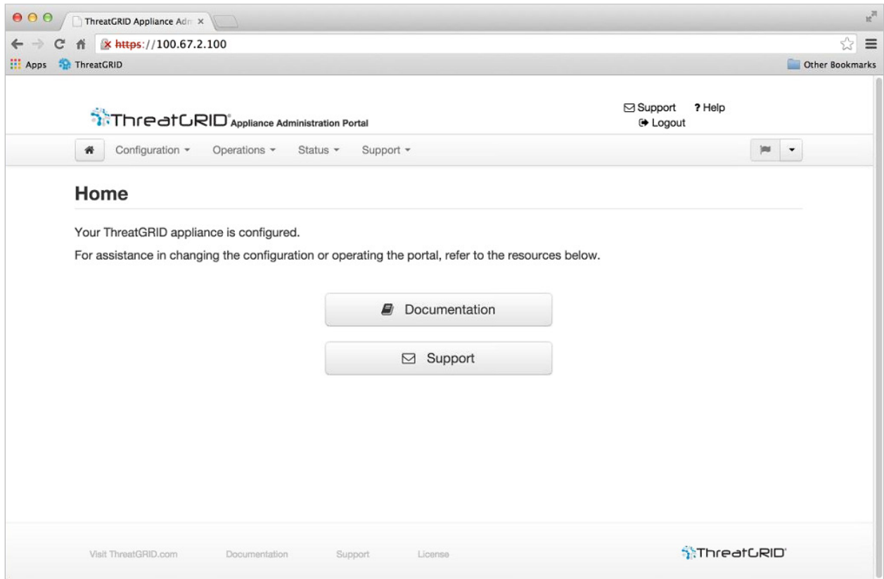
그림 23 - 어플라이언스가 구성됨
