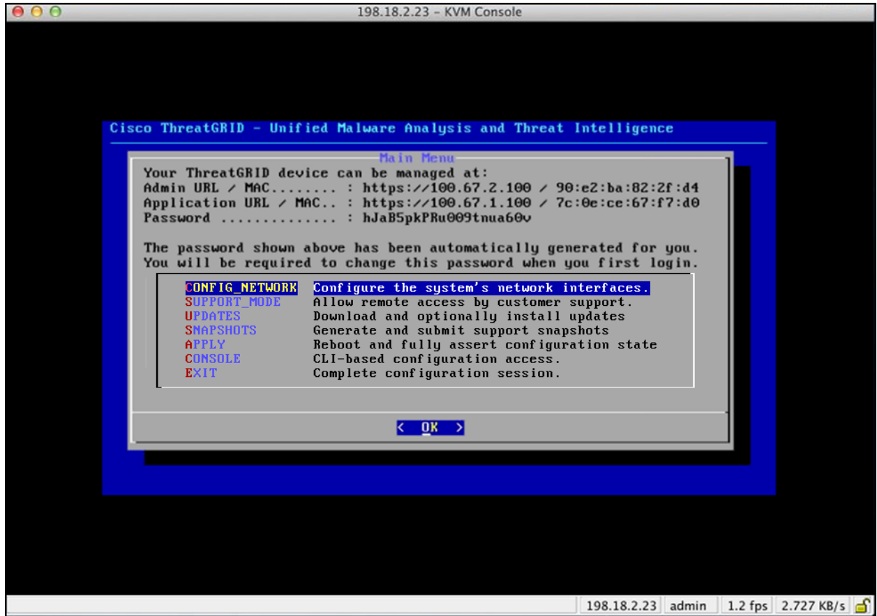
그림 13 - IP 주소
