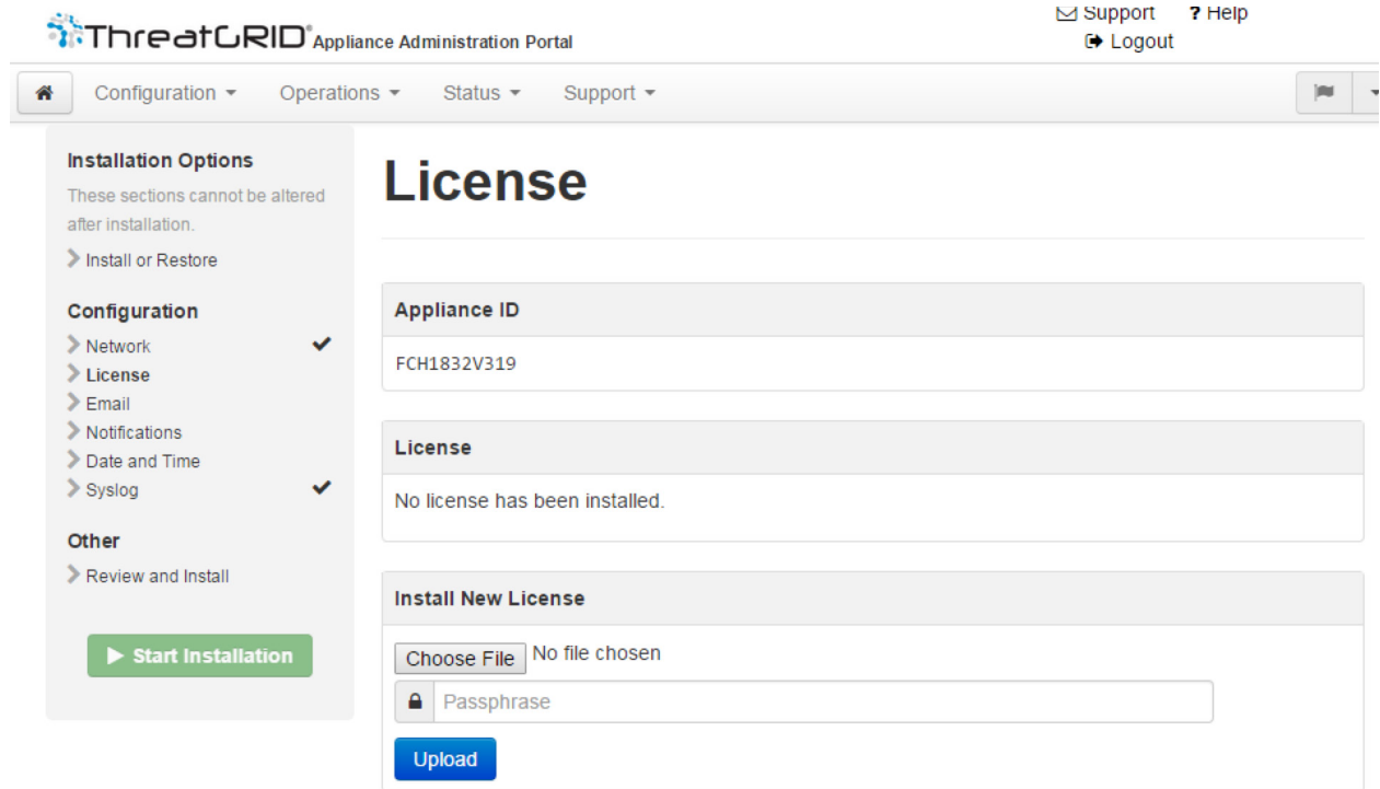
그림 17 - 라이선스 페이지
