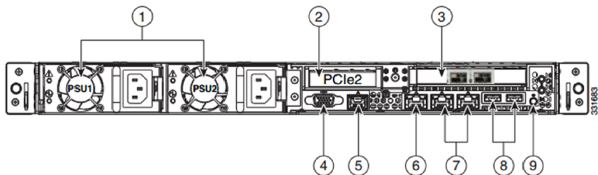
图 4 - Cisco UCS C220 M3 后视图详细信息
