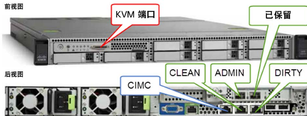
图 3 - Cisco UCS C220 M3 SFF 机架式服务器
