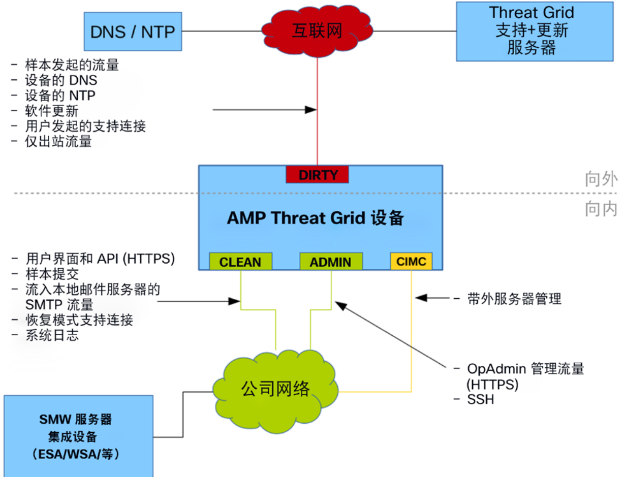
图 5 - 网络接口设置图
