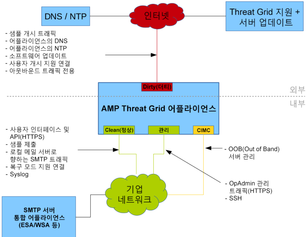
그림 5 - 네트워크 인터페이스 설정 다이어그램
