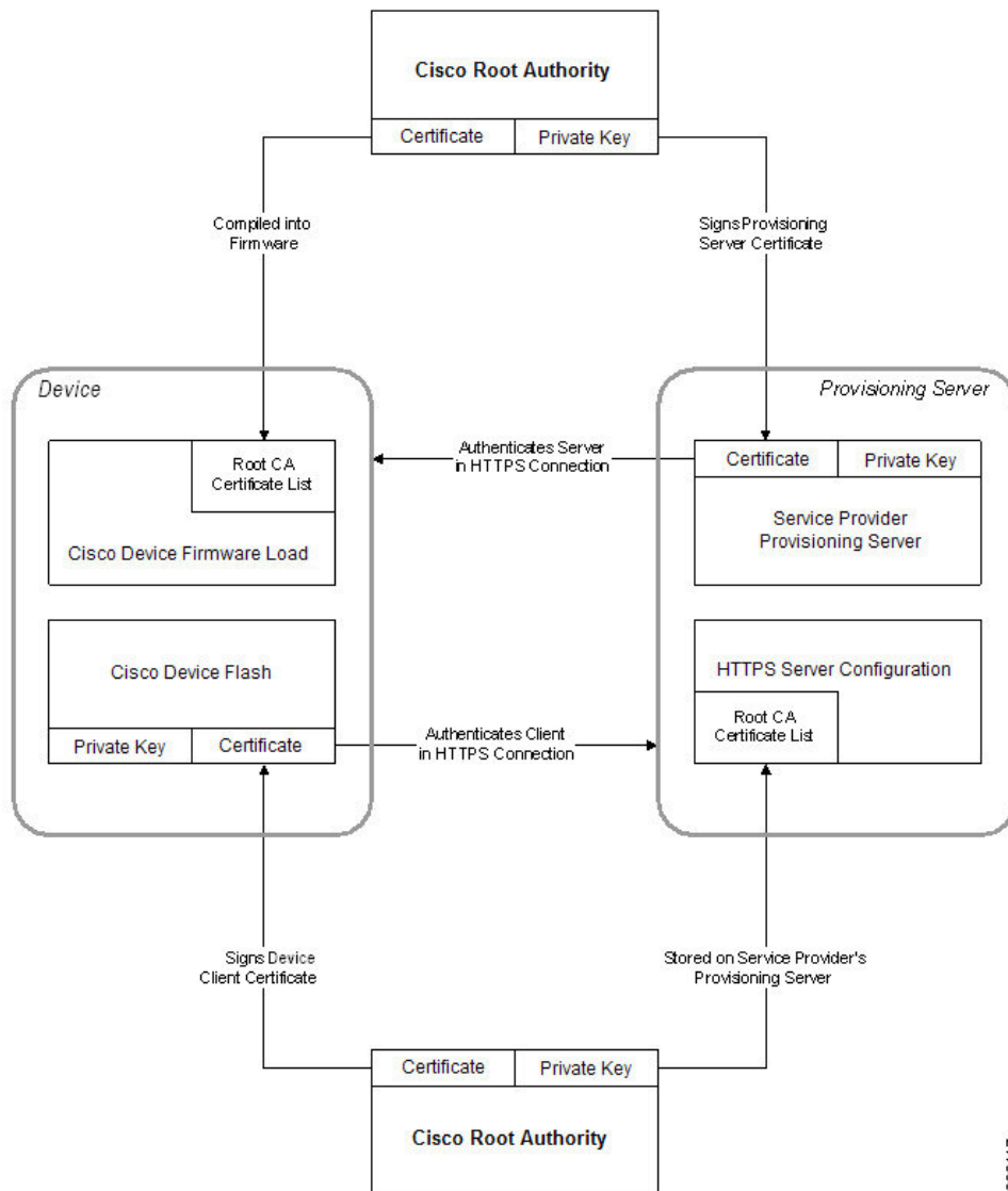
Figura 7: Fluxo de Autoridade de Certificação
