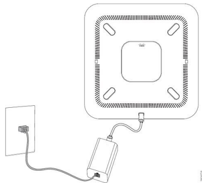
Σχήμα 3: Υλοποίηση Non-PoE
