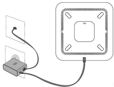
Σχήμα 3: Υλοποίηση Non-PoE
