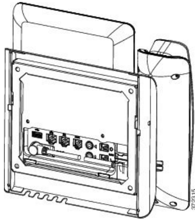
Figura 9: Vista trasera del kit para montaje en pared instalado en el teléfono
