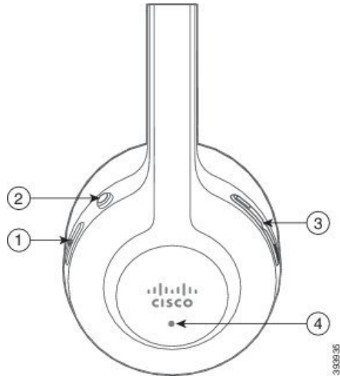
Figura 4: Botones de los auriculares Cisco 561 y 562
