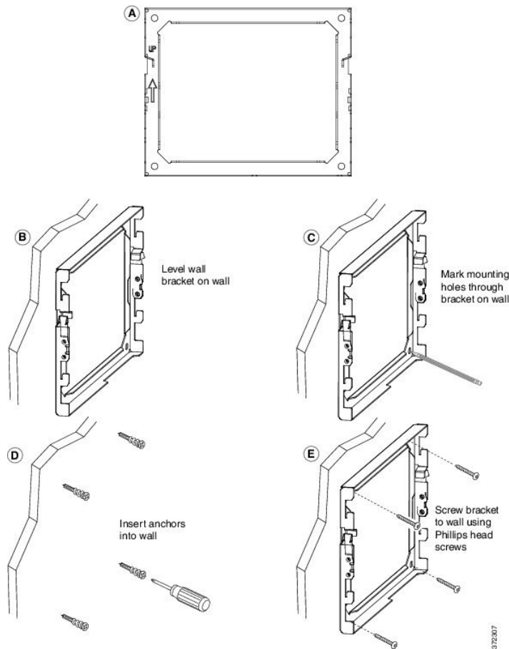
Figura 11: Instalación de la abrazadera
