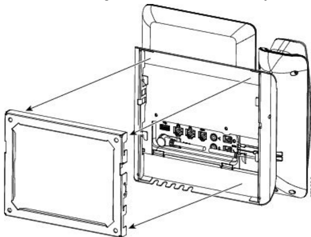
Figura 14: Acoplamiento del teléfono a la abrazadera de pared
