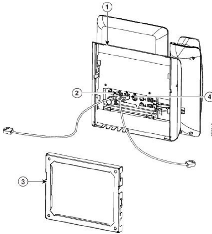
Σχήμα 13: Σύνδεση καλωδίων
