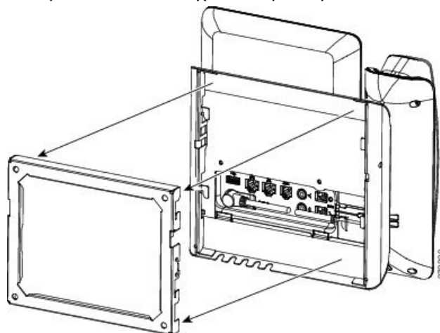
Σχήμα 14: Σύνδεση τηλεφώνου στο στήριγμα τοίχου
