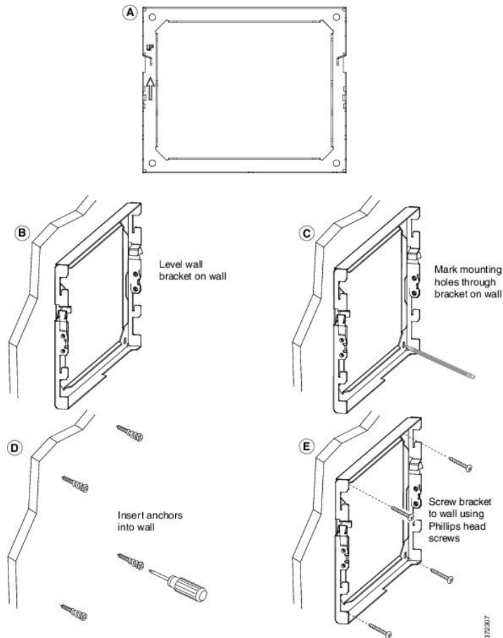
Σχήμα 11: Εγκατάσταση βραχίονα
