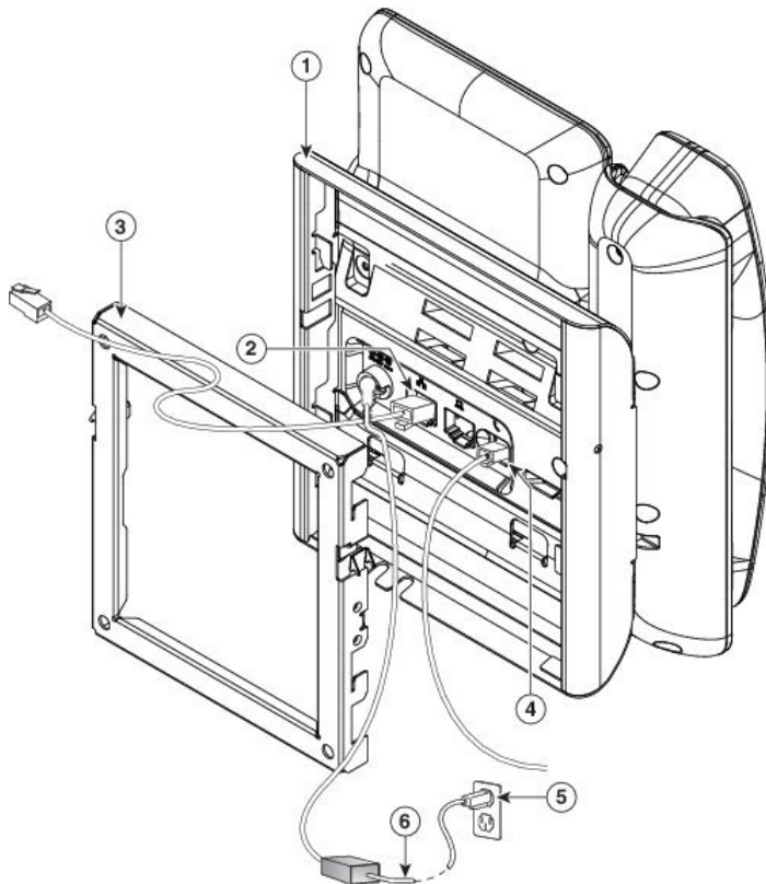
Figuur 7: Snoeren bevestigen
