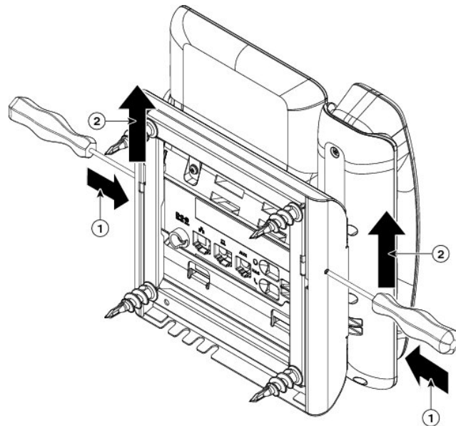
Figuur 19: Ontgrendel de nokjes
