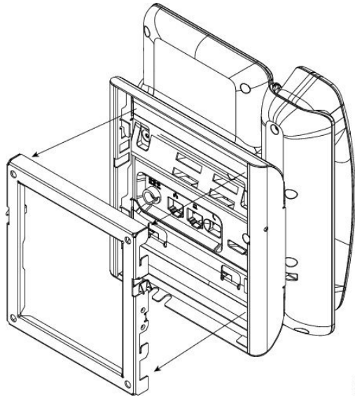
Figuur 8: Bevestiging telefoon op wandsteun
