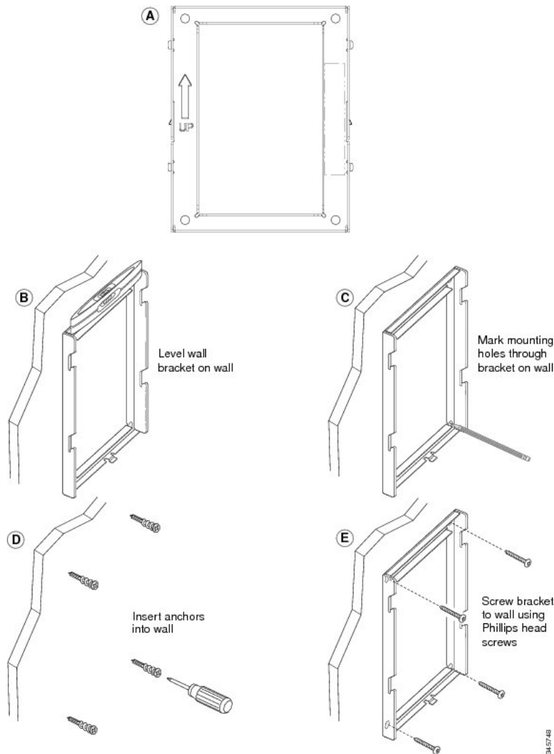
Figuur 5: Steun installeren
