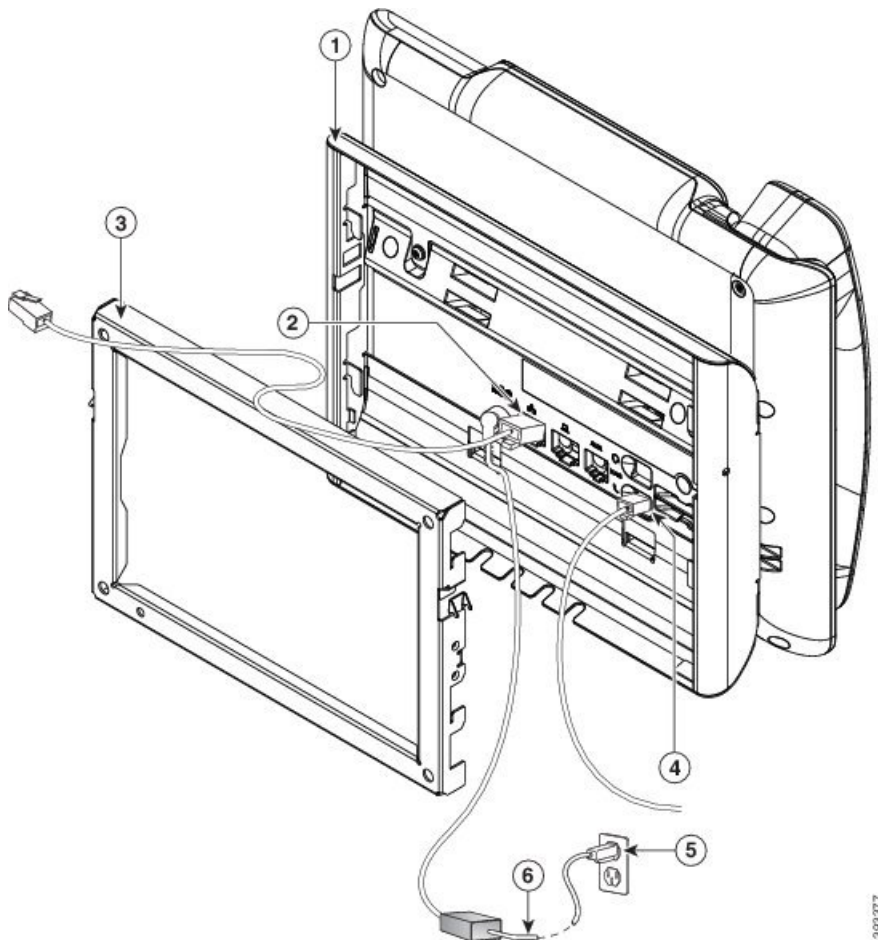
Figuur 25: Snoeren bevestigen
