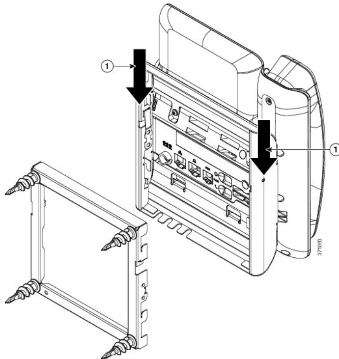
Figuur 18: Locatie nokje
