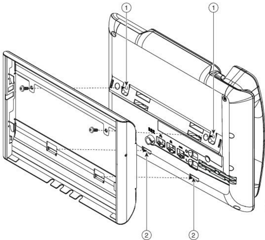
Figuur 24: Bevestiging telefoonsteun
