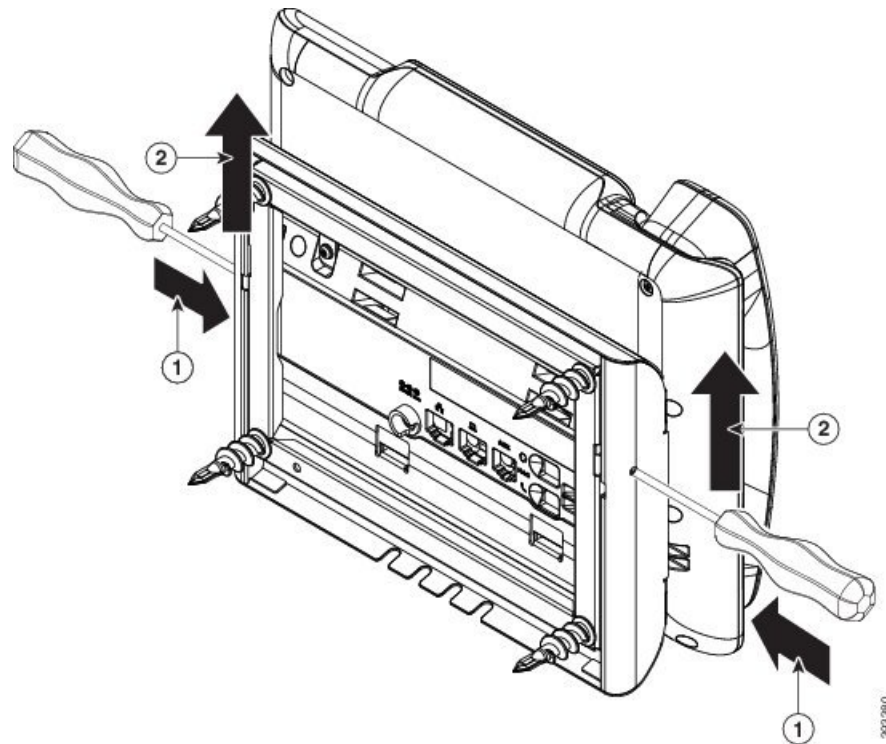
Figuur 28: Ontgrendel de nokjes
