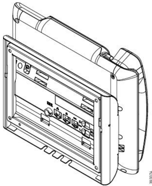
Figuur 21: Achteraanzicht van ADA niet-vergrendelbare wandmontageset op telefoon
