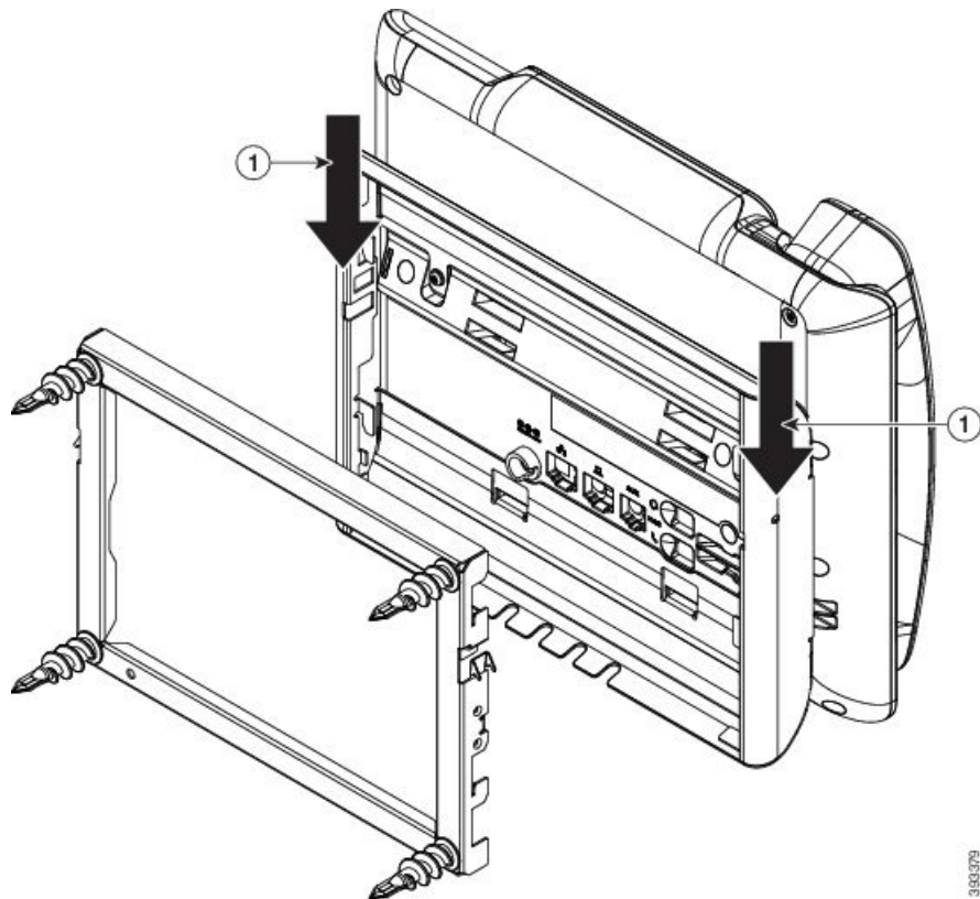
Figuur 27: Locatie nokje
