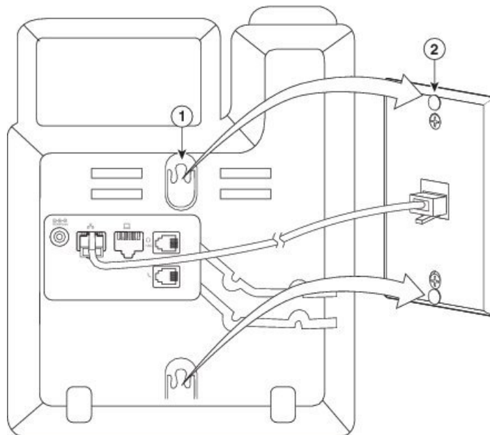
Figur 9. Monteringshål
