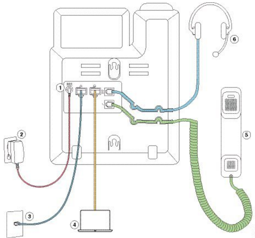
Figur 2. Cisco IP Phone 6821 multiplattformstelefoner Anslutningar
