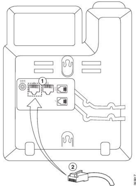
Figur 7. RJ45-kontakten i telefonjacket
