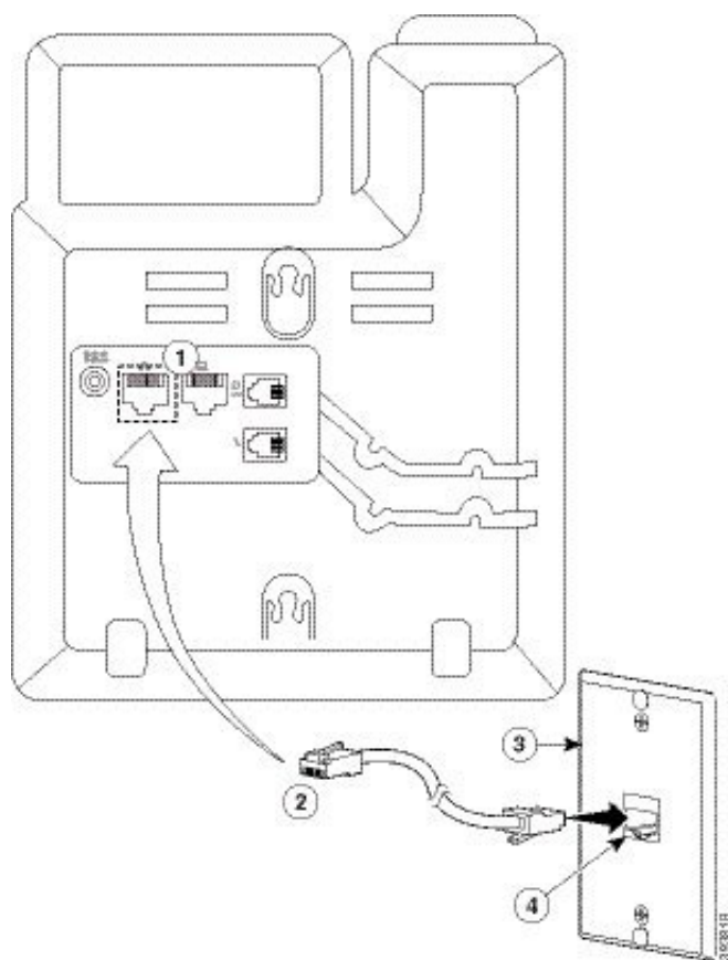
Figur 8. RJ45-kontakt i monterat väggjack
