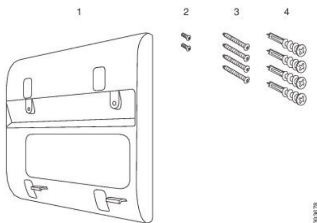
Figur 5. Väggmonteringsats för Cisco IP Phone 6800-seriens multiplattformstelefoner
