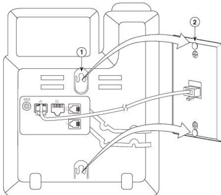
Figuur 9: Montagegaten
