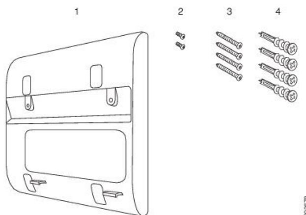
Figuur 5: Wandmontageset voor de Cisco IP Phone 6800-serie voor meerdere platforms
