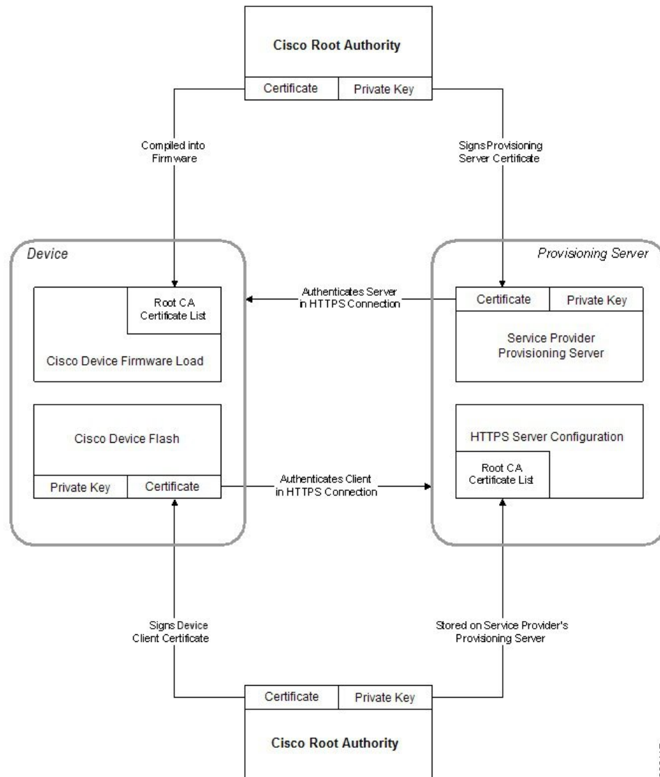
圖 6: Certificate Authority 流程
