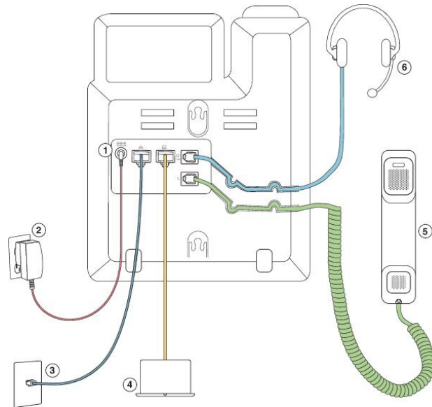
Figura 2: Teléfonos multiplataforma de Cisco IP Phone 6821 Conexiones
