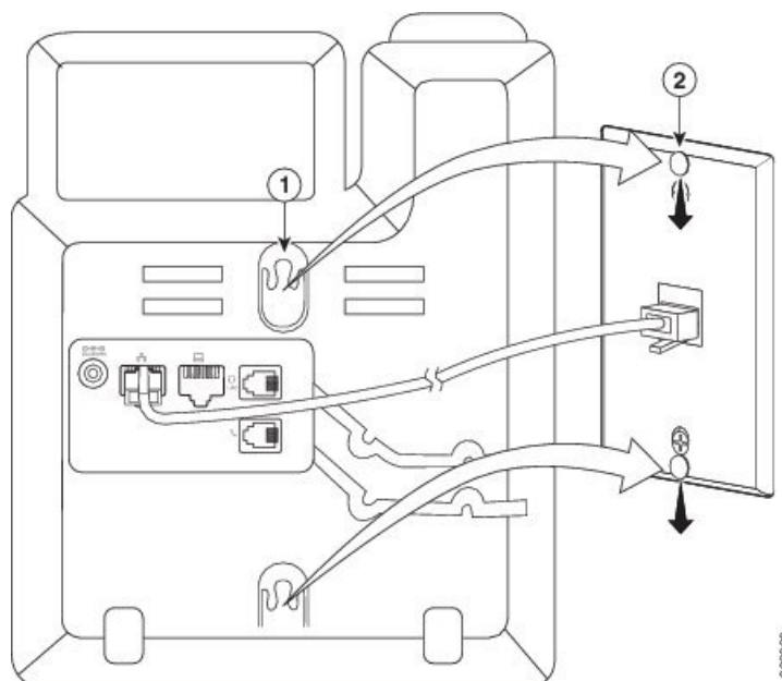
Figura 10: Deslizamiento del teléfono IP
