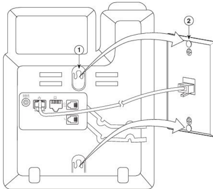
Figura 9: Orificios de montaje
