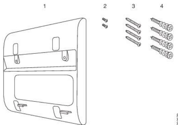
Figura 5: Kit de montaje en pared para Teléfonos IP multiplataforma de la serie 6800 de Cisco
