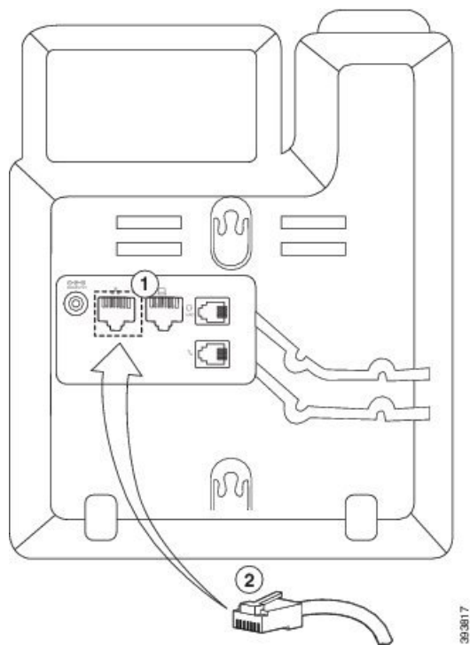
图 7: RJ45 连接器插入电话插孔
