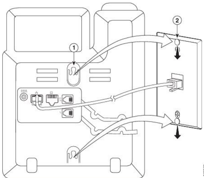
图 10: 滑动 IP Phone
