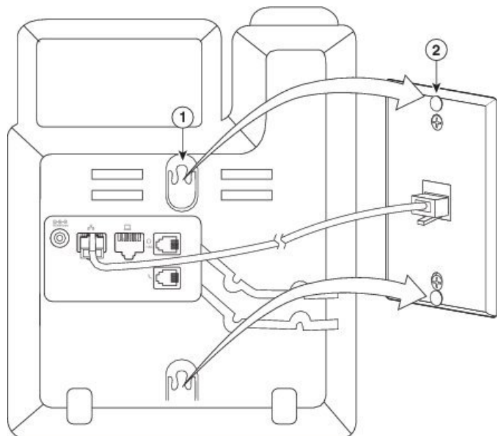
图 9: 安装孔
