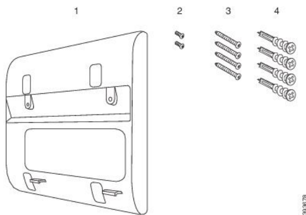
图 5: Cisco IP Phone 6800 系列多平台电话壁挂式套件
