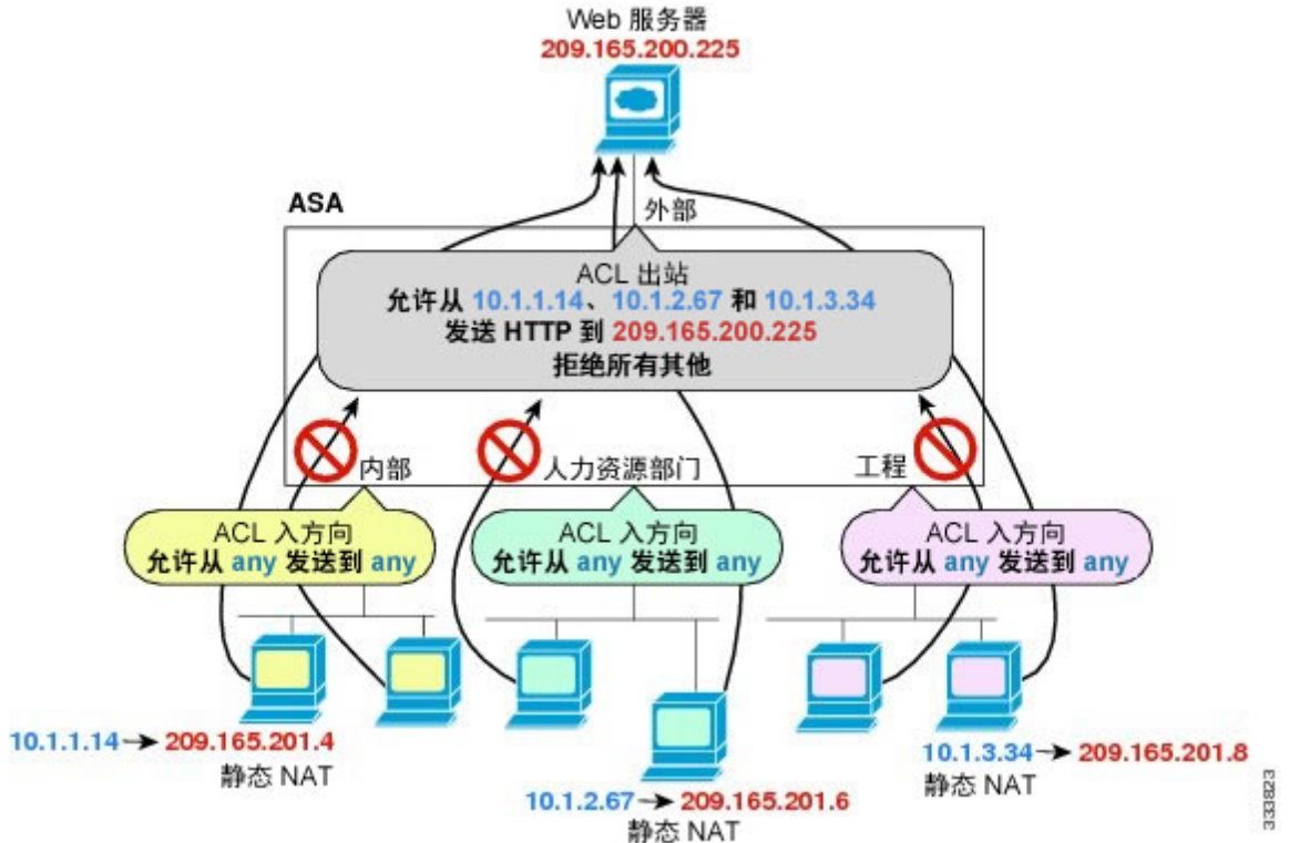
图 2: 出站 ACL
