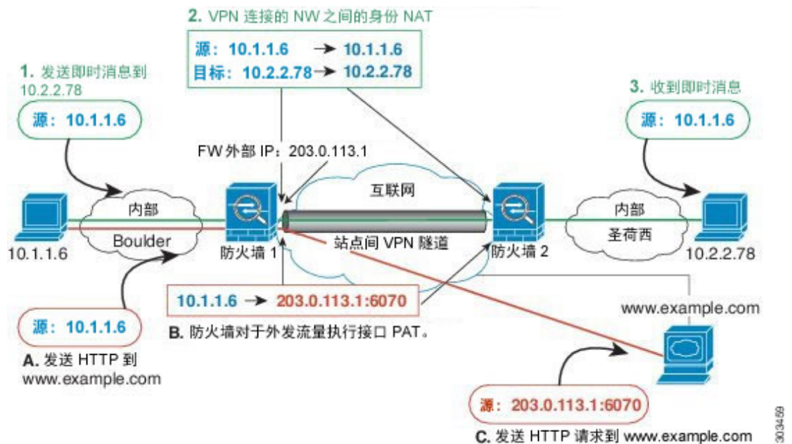
图 41: 用于站点到站点 VPN 的接口 PAT 和身份 NAT
