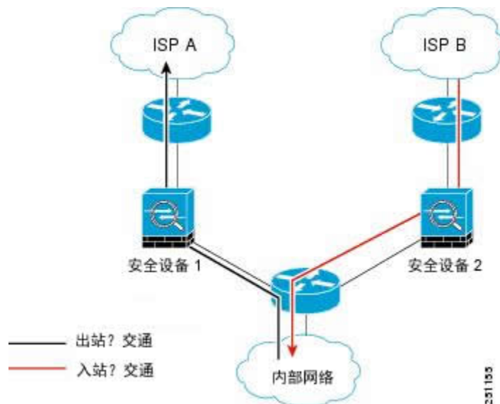
图 52: 非对称路由
