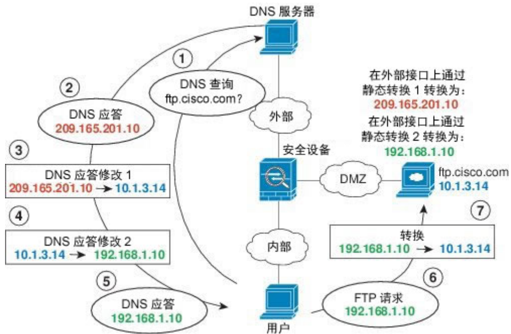
图 44: 独立网络上的 DNS 应答修改、DNS 服务器、主机和服务
