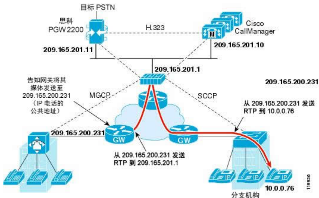
图 50: 配合使用 NAT 与 MGCP
