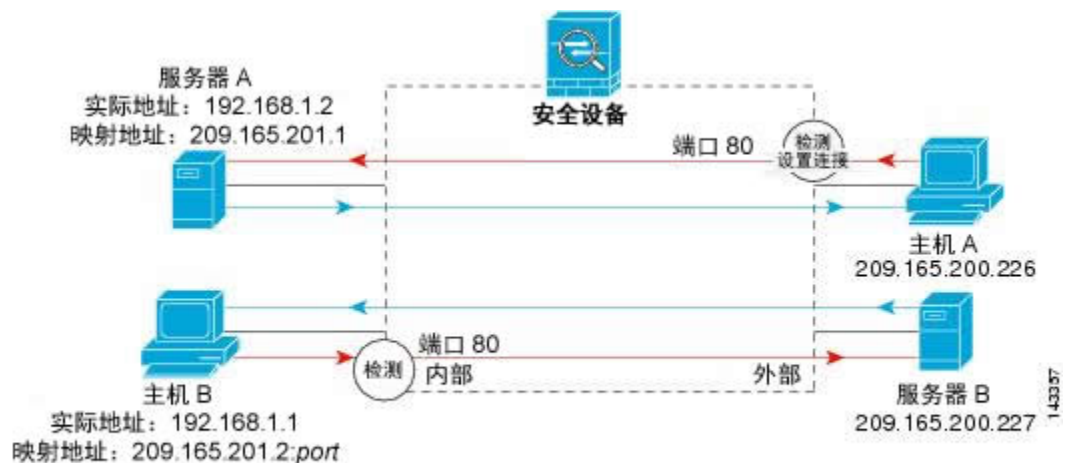
图 48: 对于特定服务器的 HTTP 检测和连接限制
