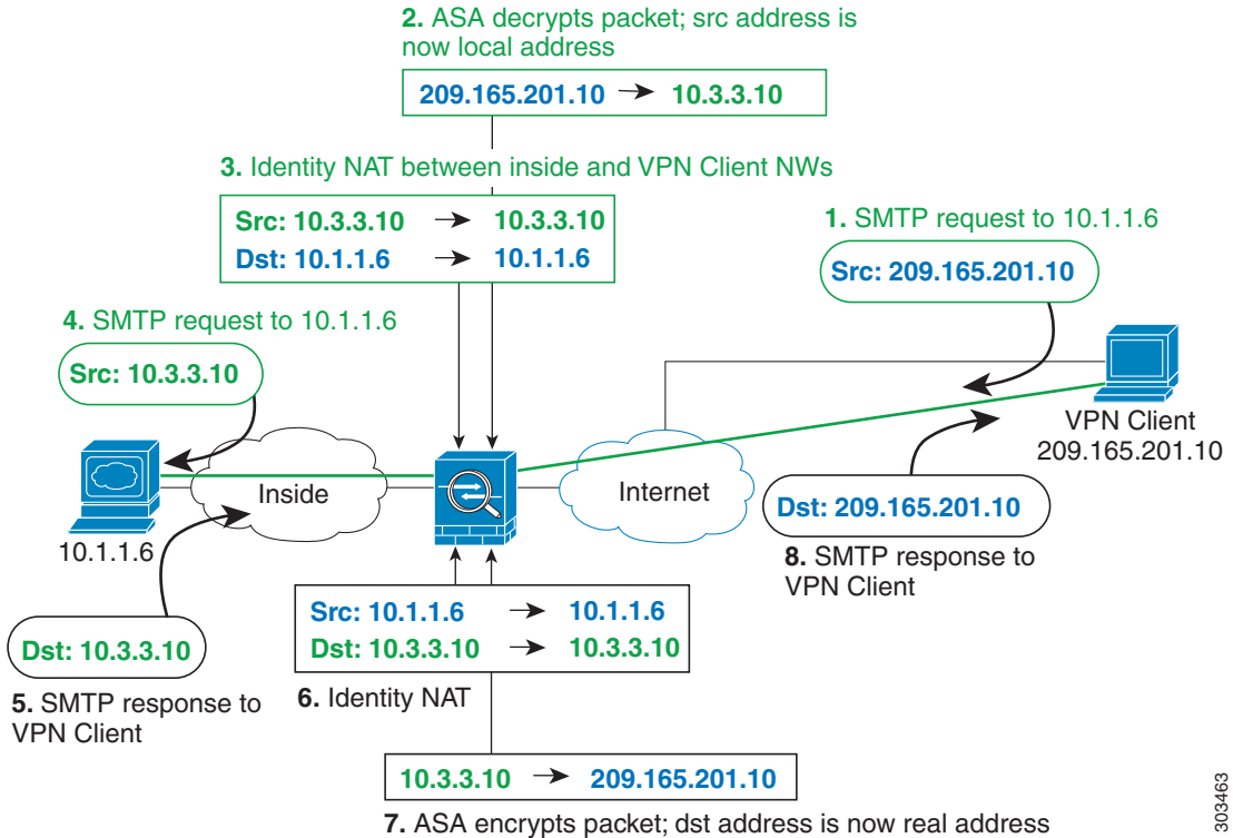
그림 5-22 VPN 클라이언트를 위한 아이덴티티 NAT
