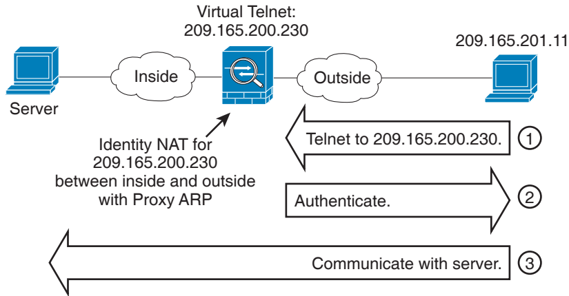
그림 5-19 프록시 ARP 및 가상 텔넷
