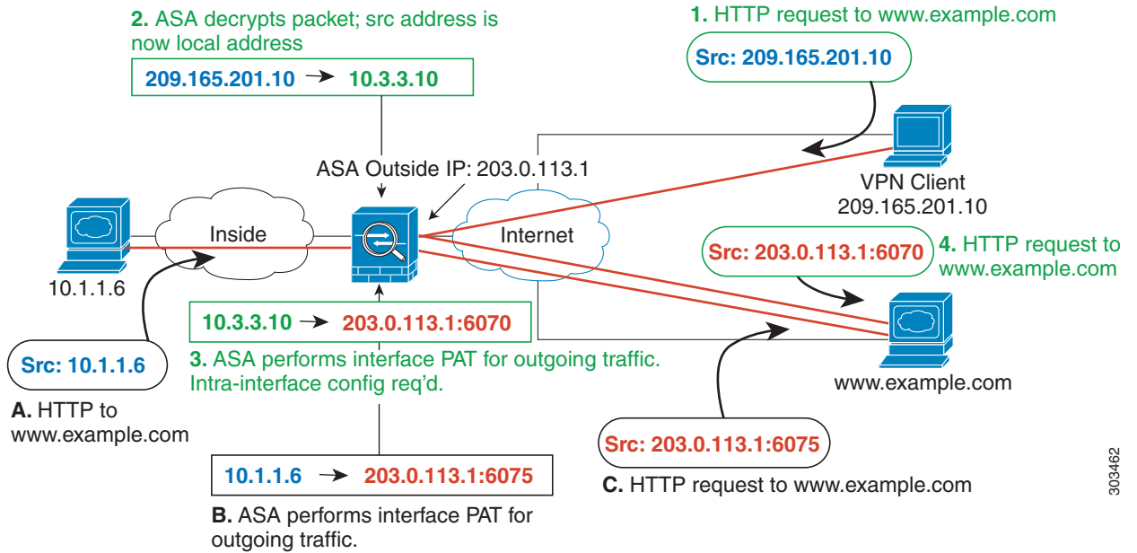
그림 5-21 인터넷 바인딩 VPN 트래픽을 위한 인터페이스 PAT(내부 인터페이스)
