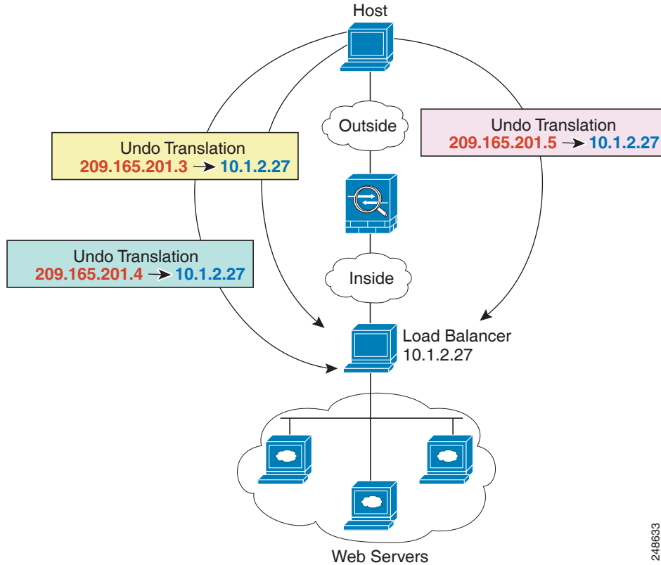
그림 6-3 내부 로드 밸런서용 일대다 고정 NAT
