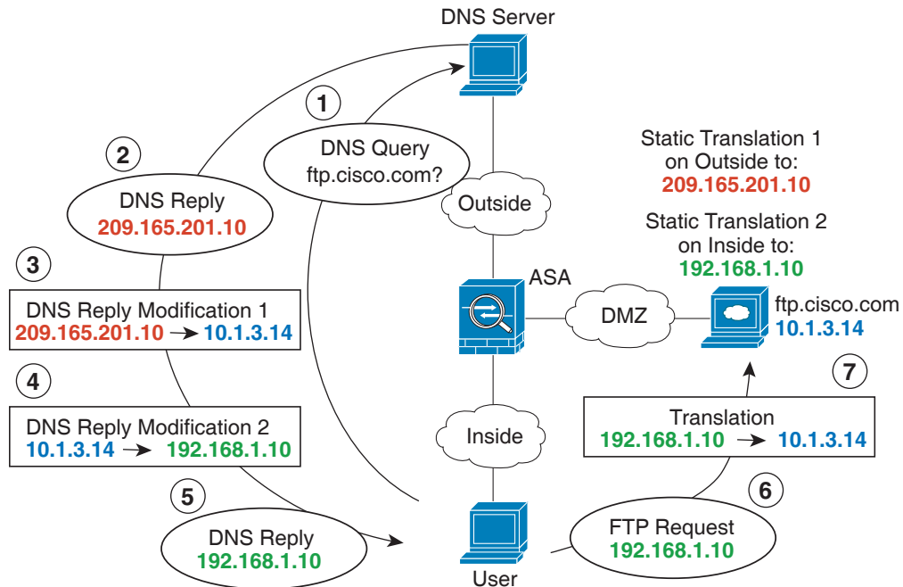
그림 5-27 DNS 회신 수정, DNS 서버, 호스트, 별도의 네트워크에 있는 서버
