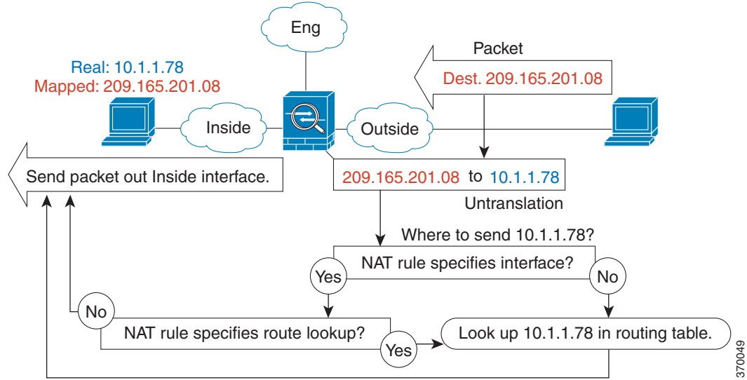
그림 5-20 라우팅된 모드 이그레스 인터페이스 선택
