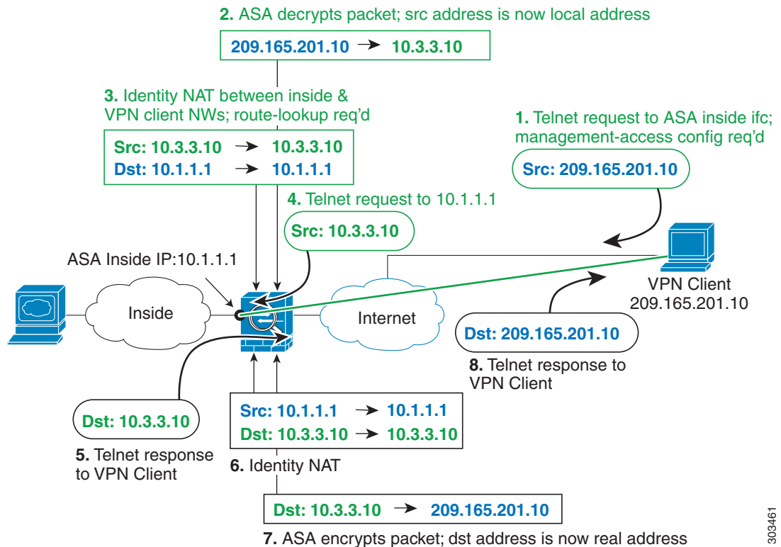
그림 5-25 VPN 관리 액세스
