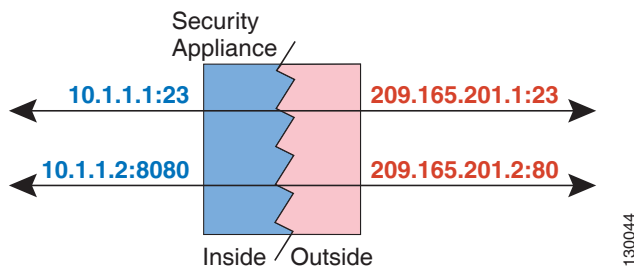
그림 5-2 일반적인 Static NAT with Port Translation 시나리오
