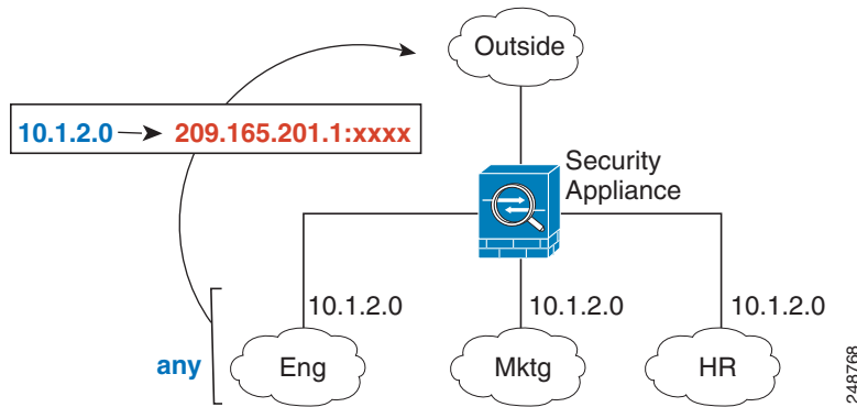
그림 5-17 임의의 인터페이스 지정
