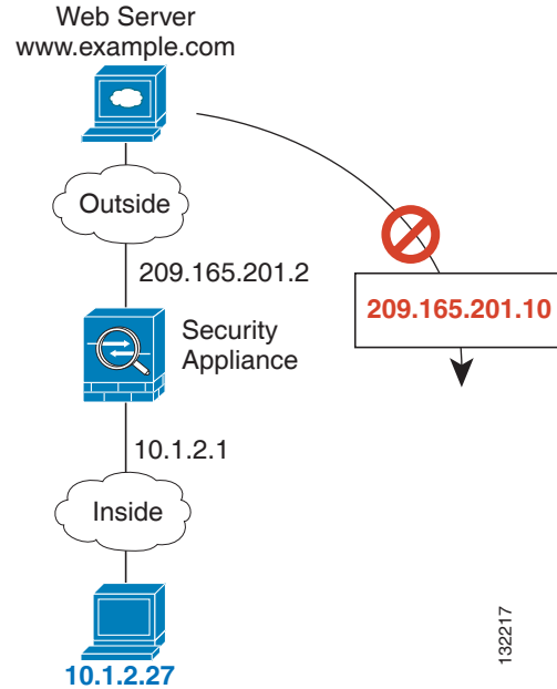
그림 5-9 매핑된 주소로 연결을 시작하려고 시도하는 원격 호스트
