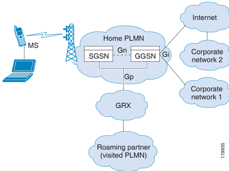
그림 12-1 GPRS 터널링 프로토콜
