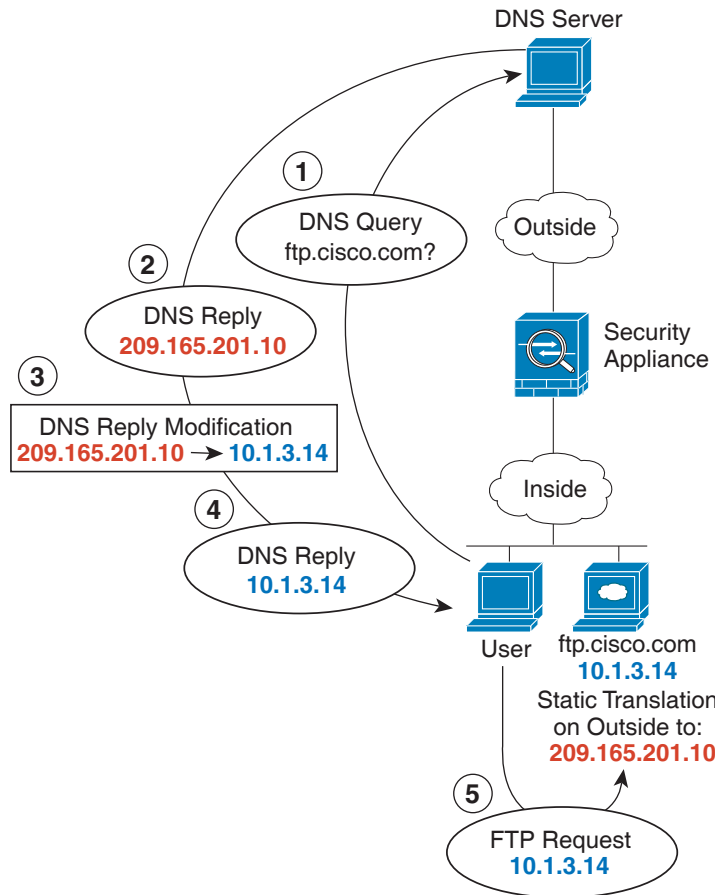
그림 5-26 DNS 회신 수정, 외부의 DNS 서버
