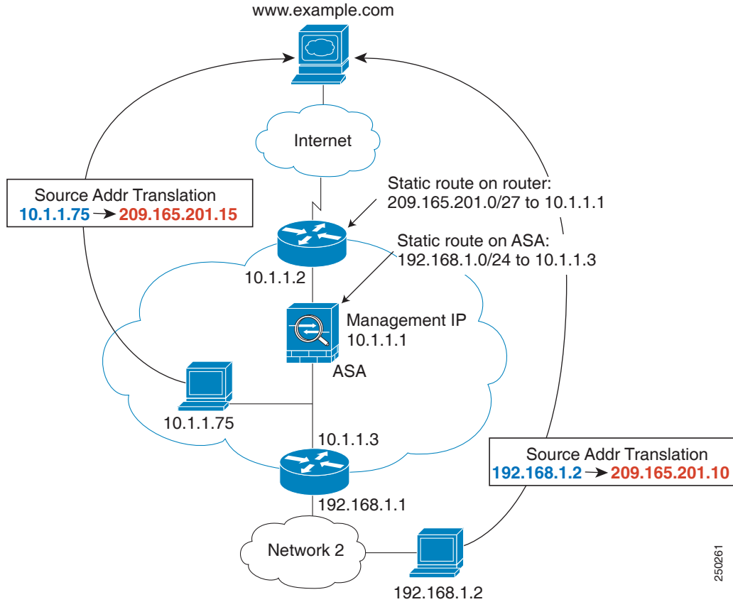
그림 5-13 NAT 예: 투명 모드
