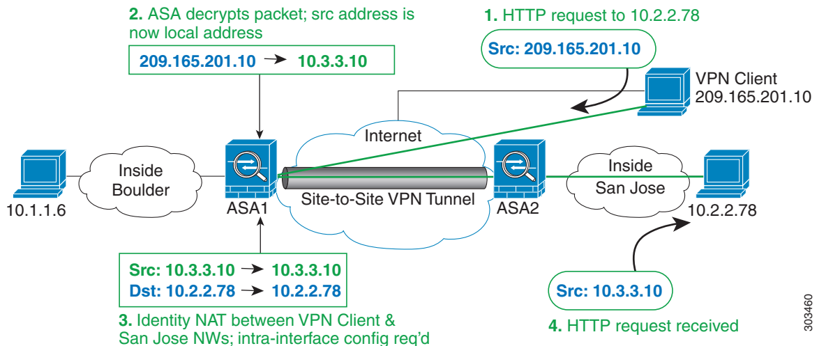
그림 5-24 Site-to-Site VPN에 대한 VPN 클라이언트 액세스
