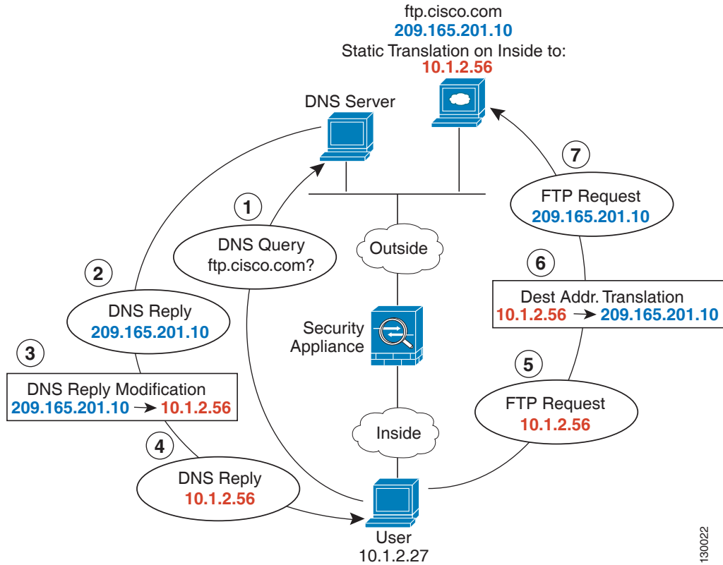
그림 6-6 외부 NAT를 사용한 DNS 회신 수정
