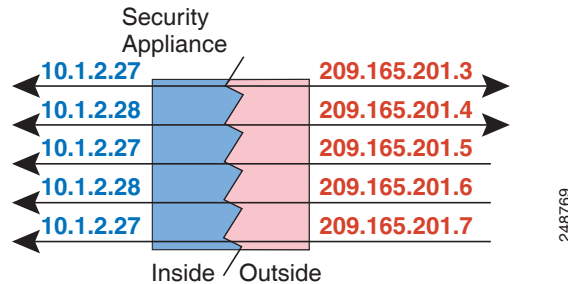
그림 5-6 소수대다수(Few-to-Many) 고정 NAT
