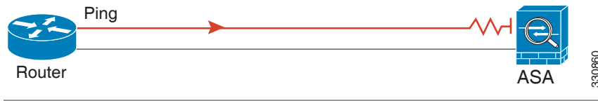
그림 15-4 ASA에 반환 경로가 없기 때문에 Ping 실패
