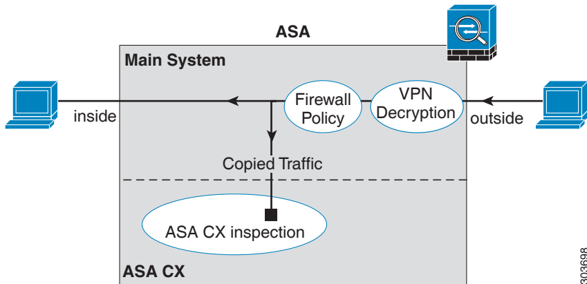
그림 19-2 ASA CX 모니터 전용
