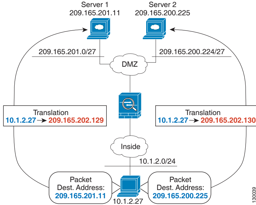
그림 5-14 서로 다른 수신 주소의 Twice NAT
