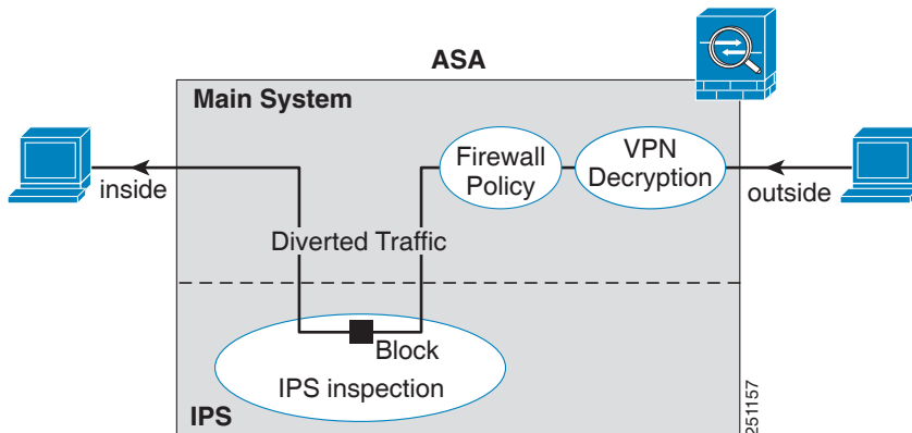
그림 20-1 ASA에서 ASA IPS 모듈 트래픽 흐름: 인라인 모드
