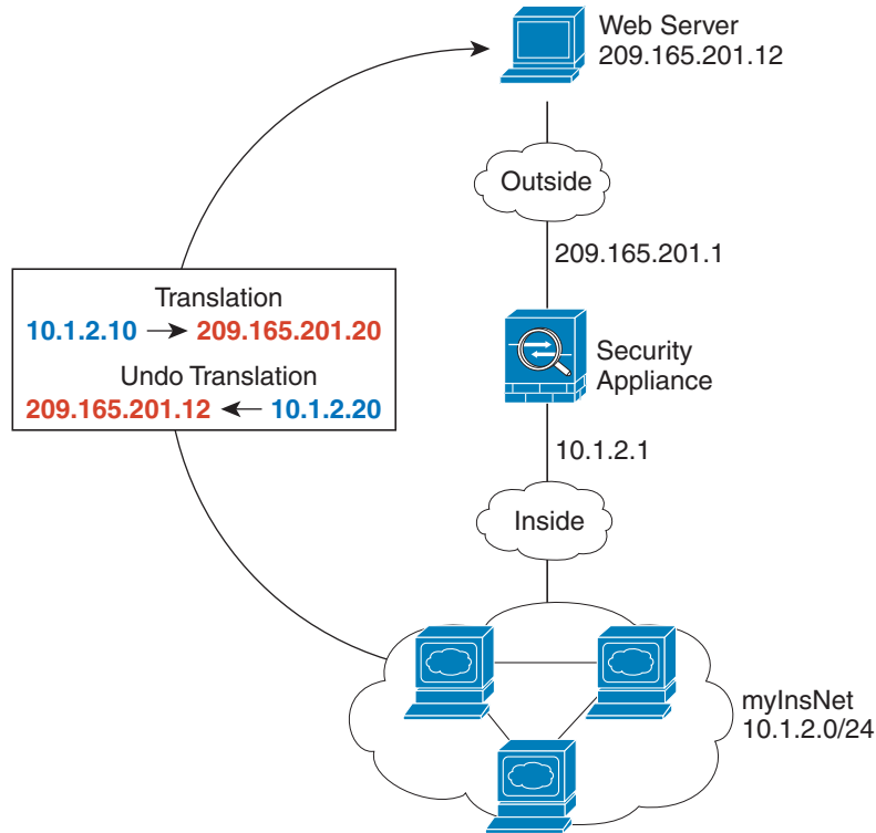
그림 6-2 내부용 동적 NAT, 외부 웹 서버용 고정 NAT
