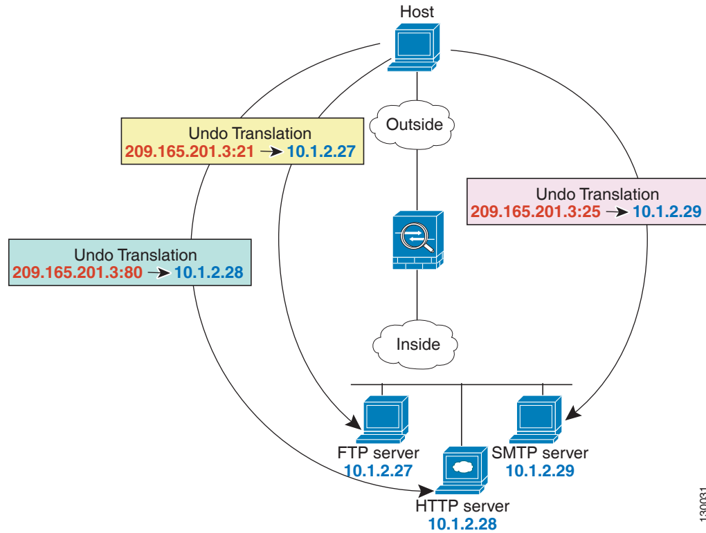
그림 5-3 Static NAT with Port Translation
