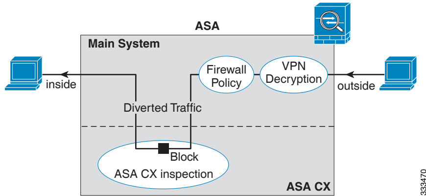
그림 19-1 ASA에서 ASA CX 모듈 트래픽 흐름
