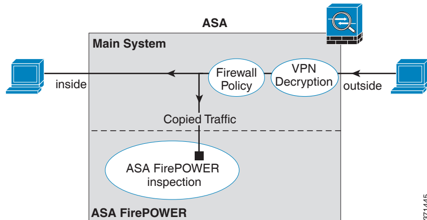
그림 18-2 ASA FirePOWER 패시브, 모니터 전용 모드
