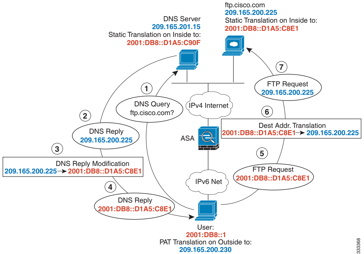
그림 6-7 외부 NAT를 사용한 DNS 회신 수정
