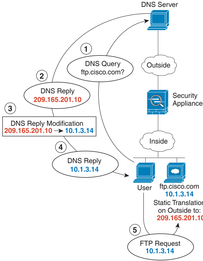
그림 6-5 DNS 회신 수정
