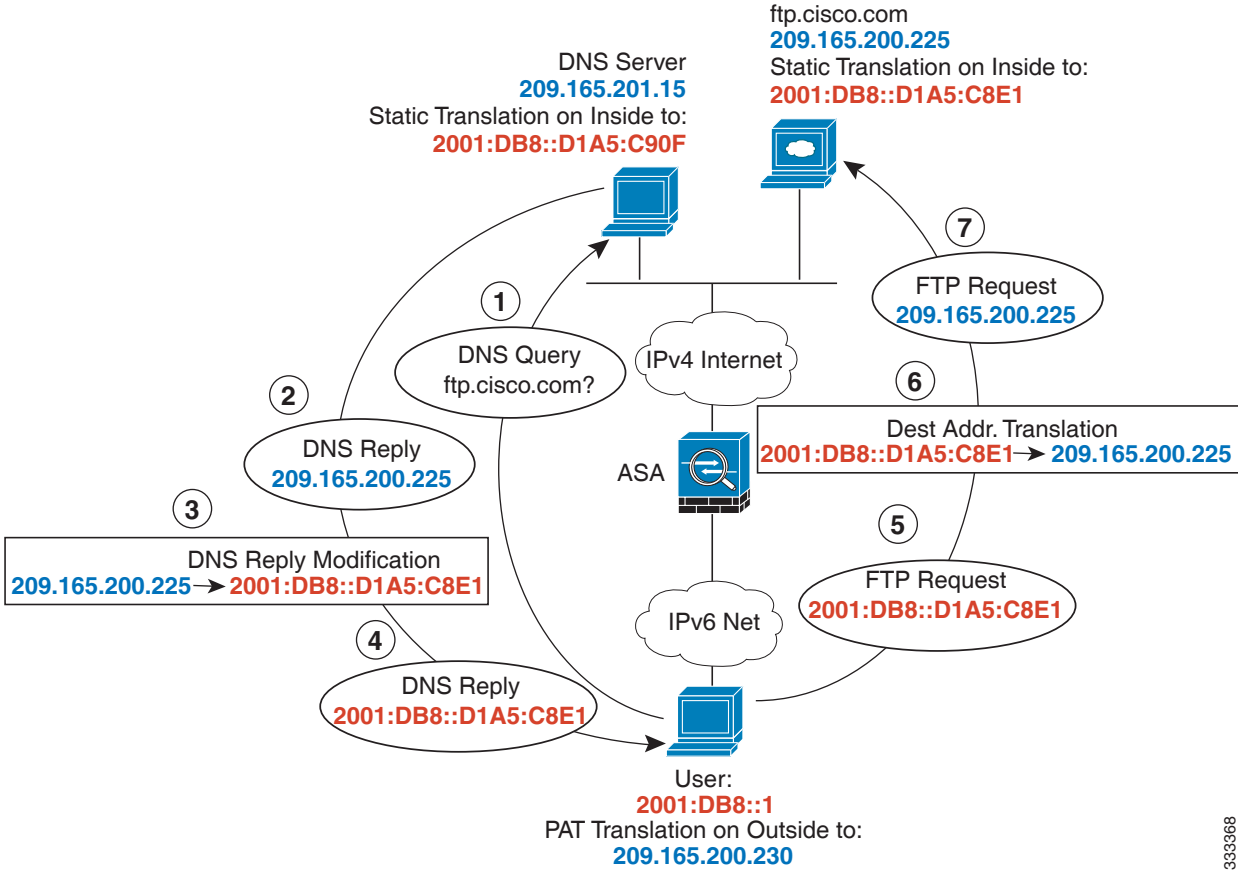
그림 5-29 외부 NAT를 사용한 DNS64 회신 수정
