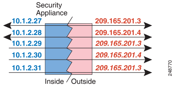
그림 5-7 다수대소수(Many-to-Few) 고정 NAT
