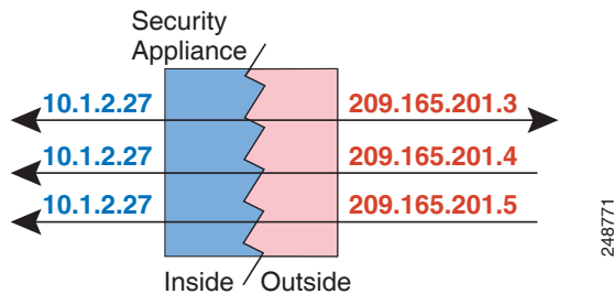
그림 5-4 일대다 고정 NAT
