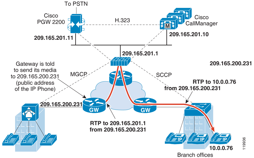
그림 10-1 MGCP와 함께 NAT 사용
