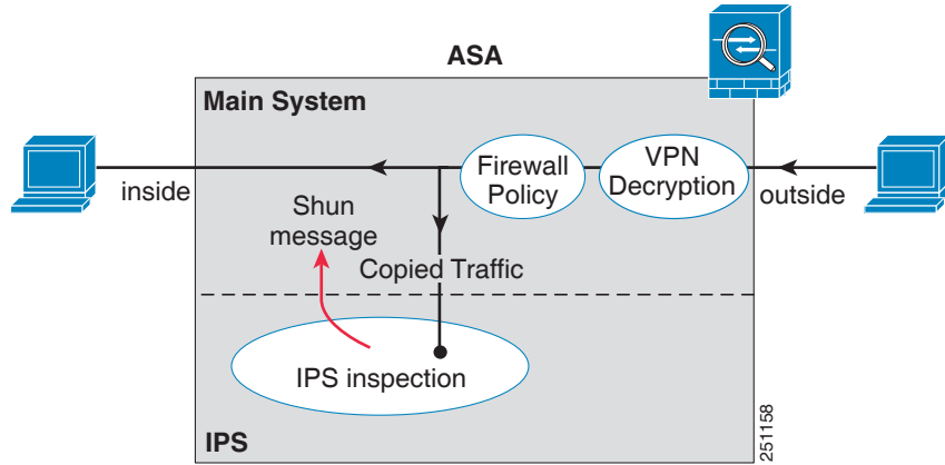
그림 20-2 ASA의 ASA IPS 모듈 트래픽 흐름: 프로미스큐어스 모드
