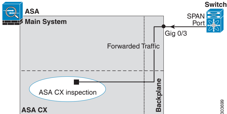
그림 19-3 ASA CX 트래픽 포워딩
