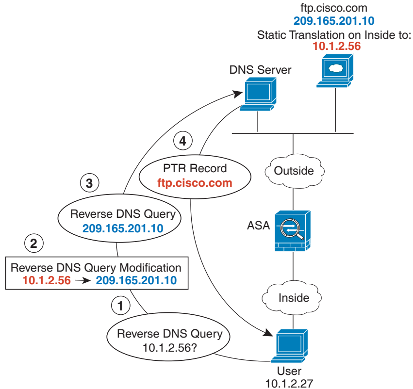
그림 5-30 PTR 수정, 호스트 네트워크의 DNS 서버
