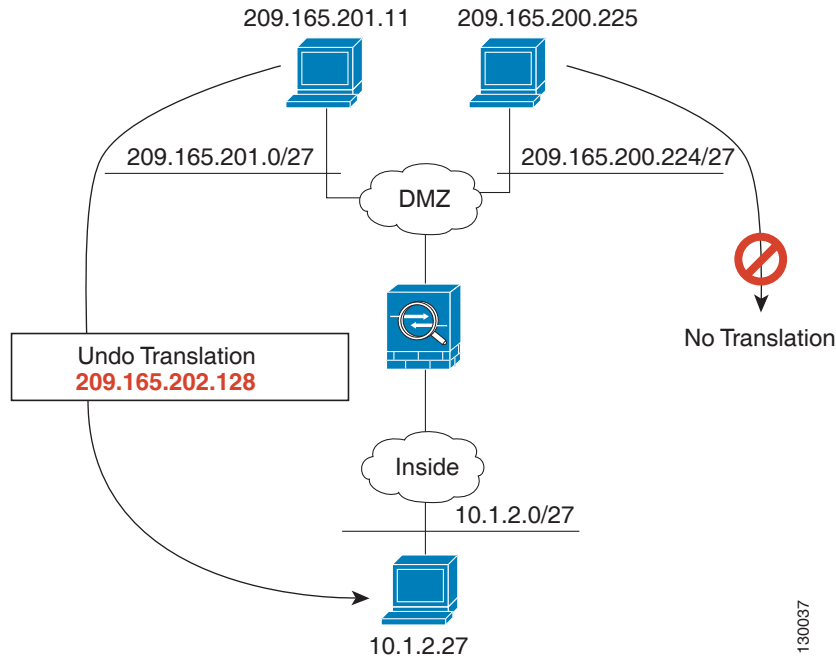
그림 5-16 수신 주소가 변환되는 Twice Static NAT
