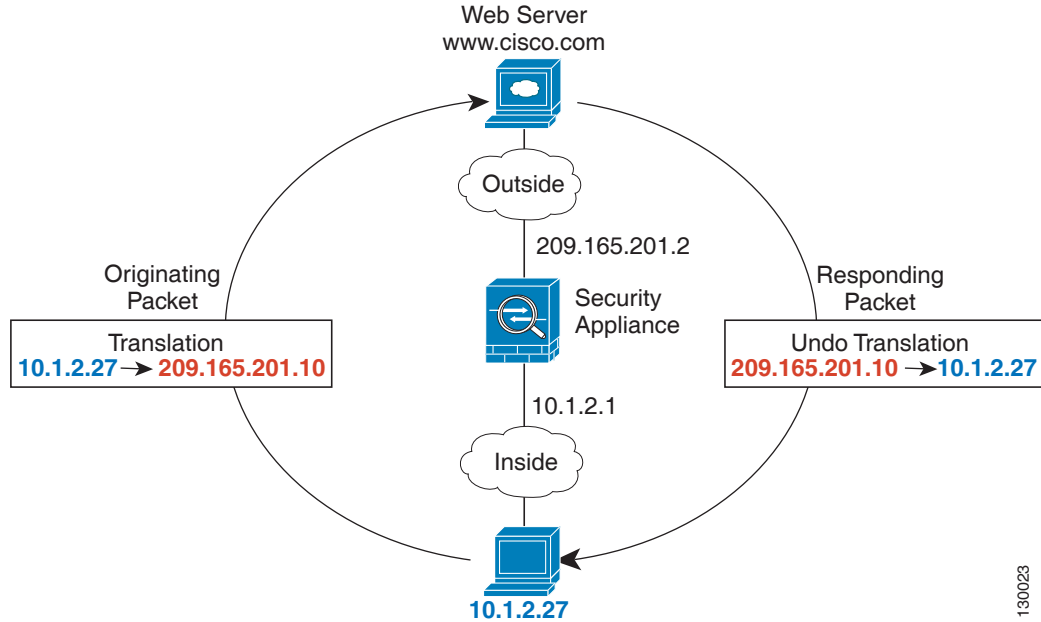
그림 5-12 NAT 예: 라우팅된 모드
