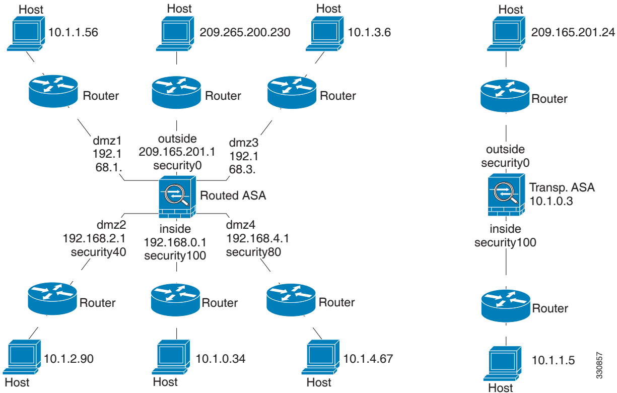
그림 15-1 인터페이스, 라우터 및 호스트가 포함된 네트워크 다이어그램
