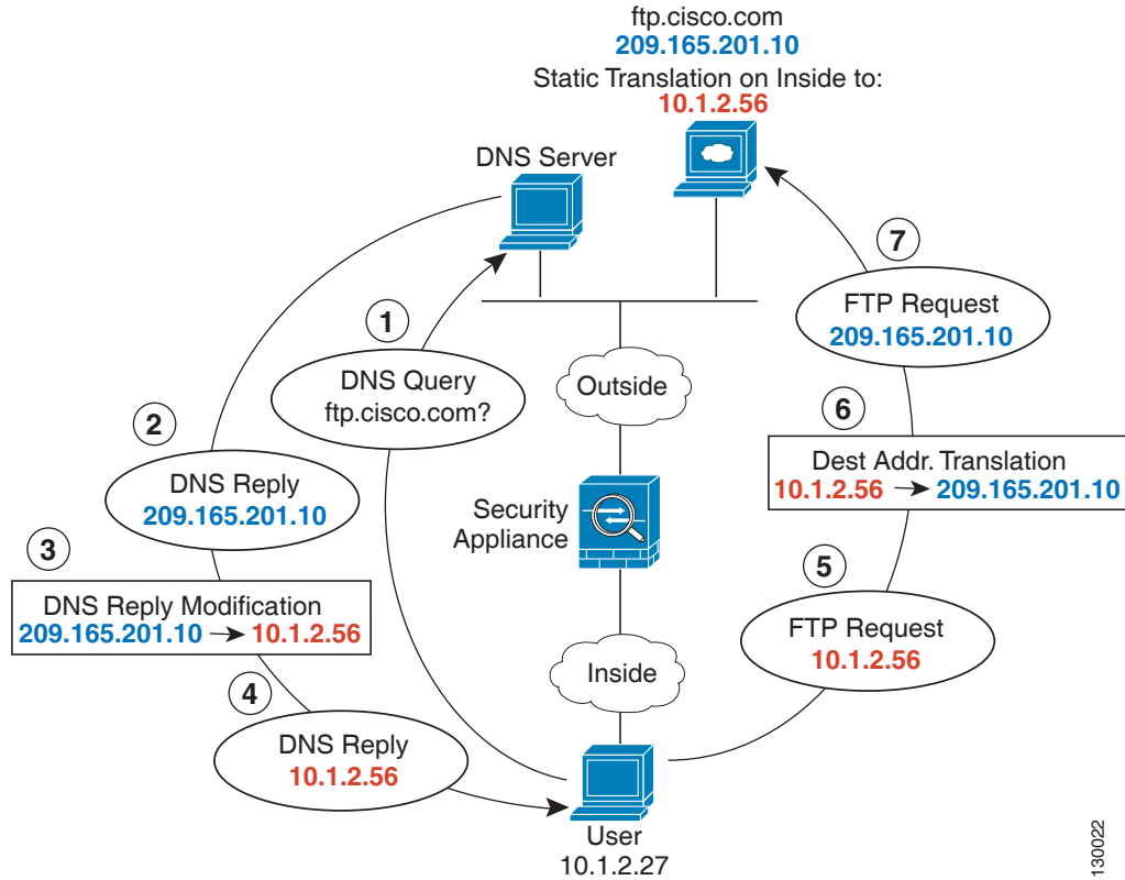
그림 5-28 DNS 회신 수정, 호스트 네트워크의 DNS 서버
