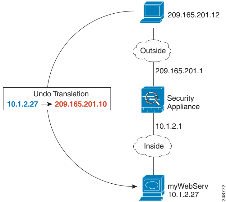
그림 6-1 내부 웹 서버에 대한 고정 NAT
