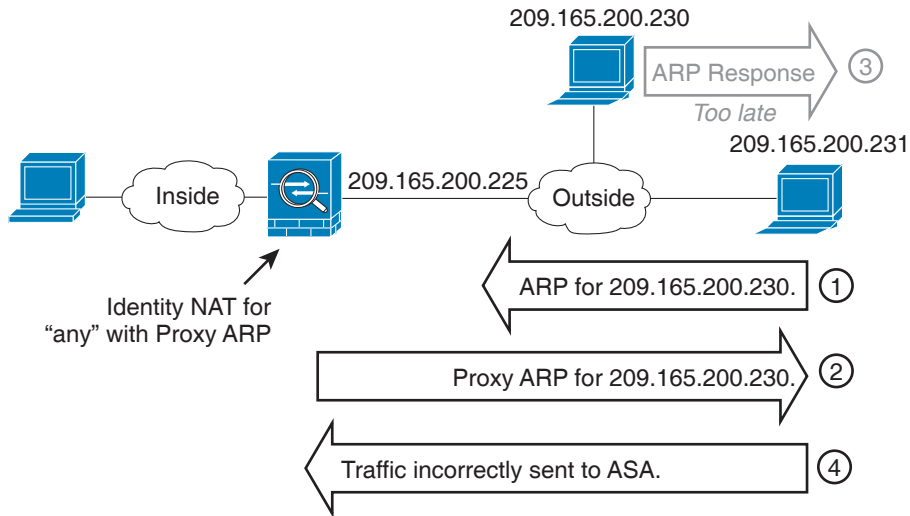
그림 5-18 아이덴티티 NAT의 프록시 ARP 문제
