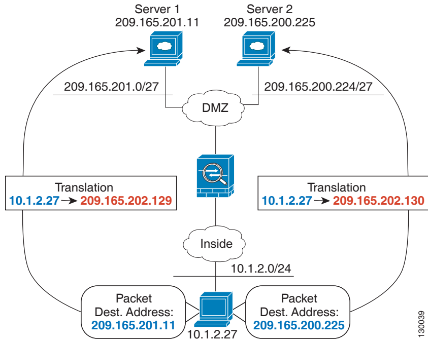
그림 7-1 서로 다른 수신 주소의 Twice NAT
