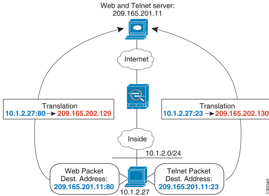
그림 5-15 서로 다른 목적지 포트의 Twice NAT
