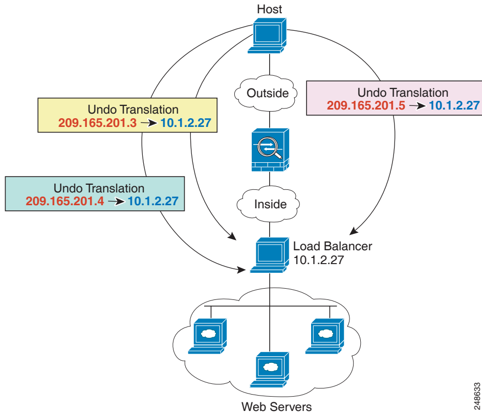
그림 5-5 일대다 고정 NAT 예
