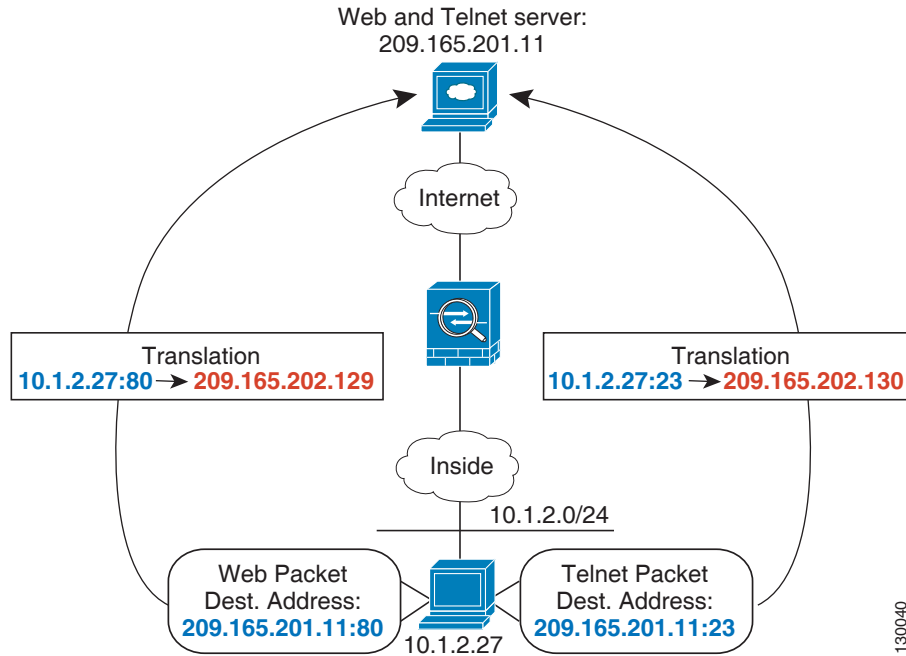
그림 7-2 서로 다른 목적지 포트의 Twice NAT
