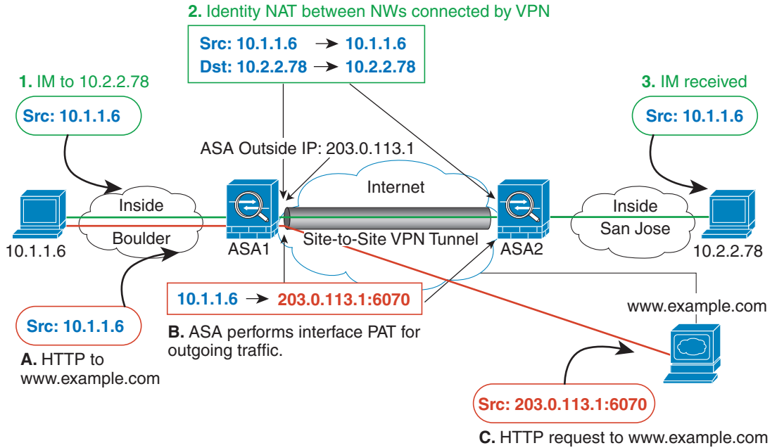
그림 5-23 Site-to-Site VPN을 위한 인터페이스 PAT 및 아이덴티티 NAT
