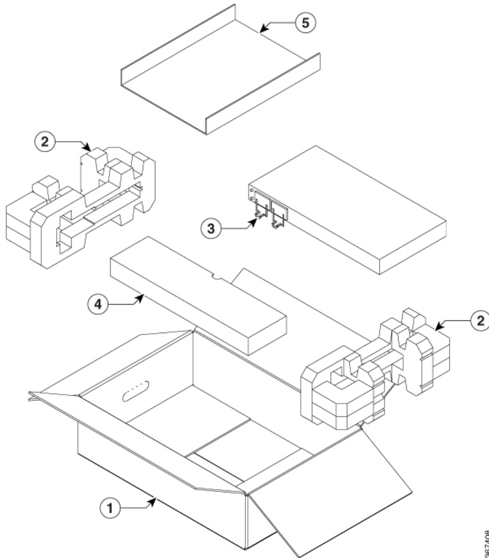
Figura 4: Embalaje de envío del router
