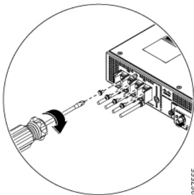
Figura 25: Fijación de los cables a la fuente de alimentación de CC
