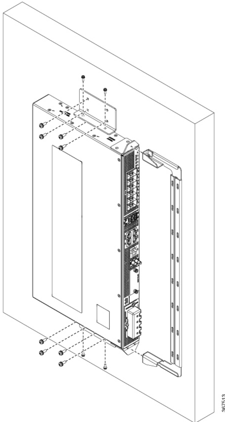
Figura 19: Montaje en pared del dispositivo
