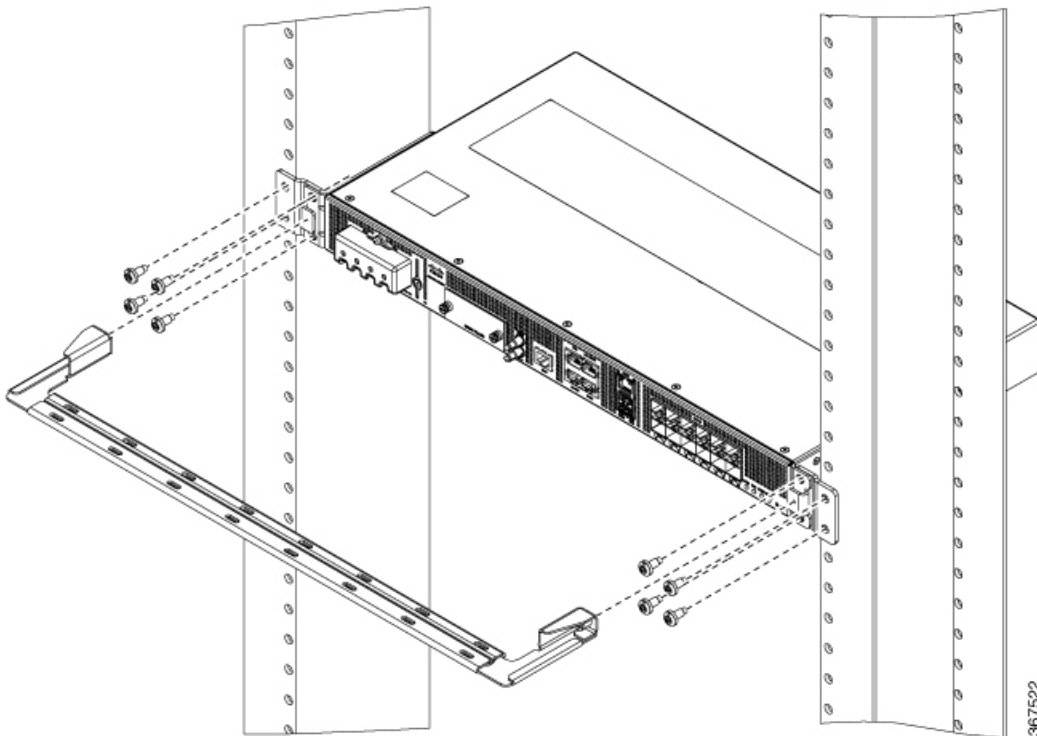
Figura 16: Dispositivo de montaje delantero con guía de cable en rack de 21 pulgadas
