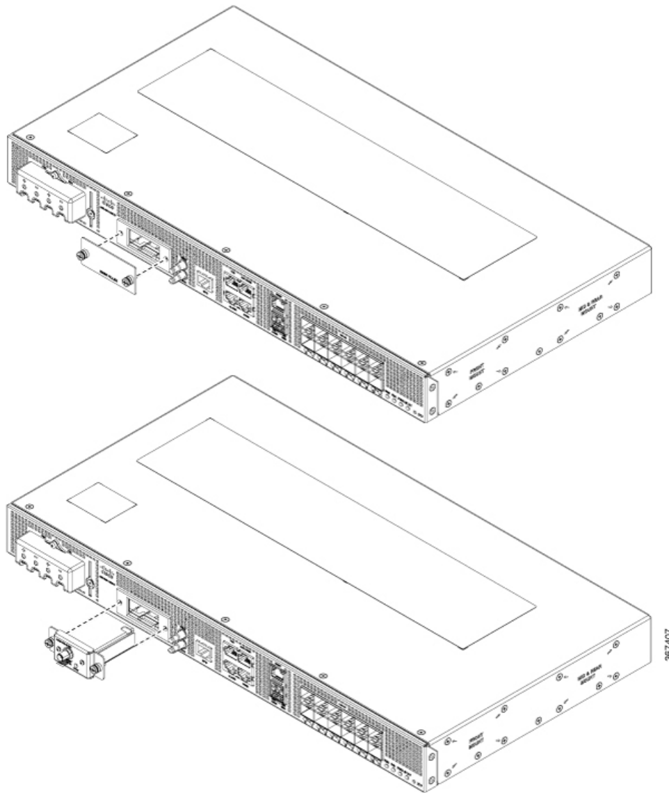
Figura 29: Instalación del módulo GNSS
