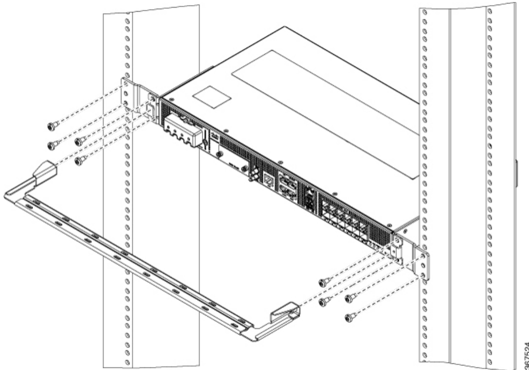
Figura 17: Dispositivo de montaje delantero con guía de cable en rack de 23 pulgadas
