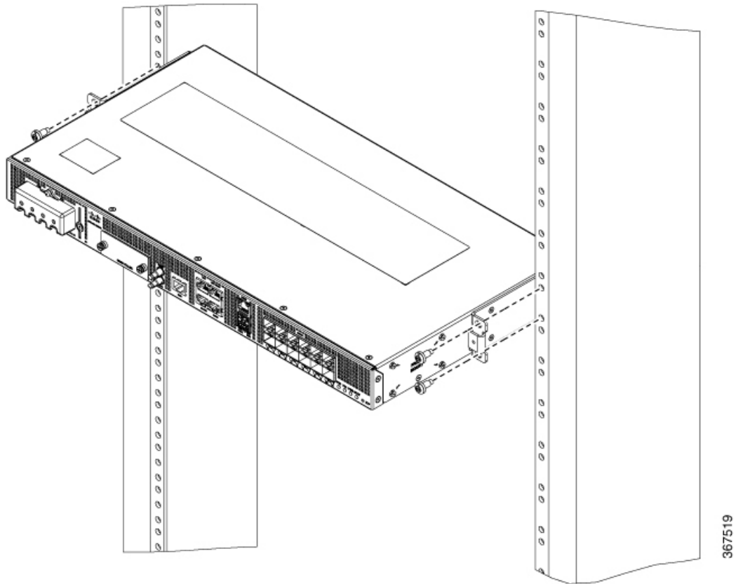
Figura 9: Configuración del dispositivo en rack de 19 pulgadas (montaje central)
