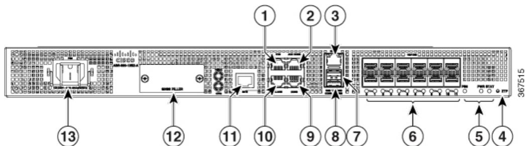
Figura 1: Vista del panel frontal del Cisco ASR-920-12SZ-A
