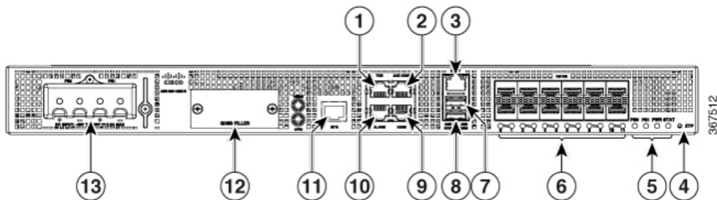
Figura 2: Vista del panel frontal del Cisco ASR-920-12SZ-D
