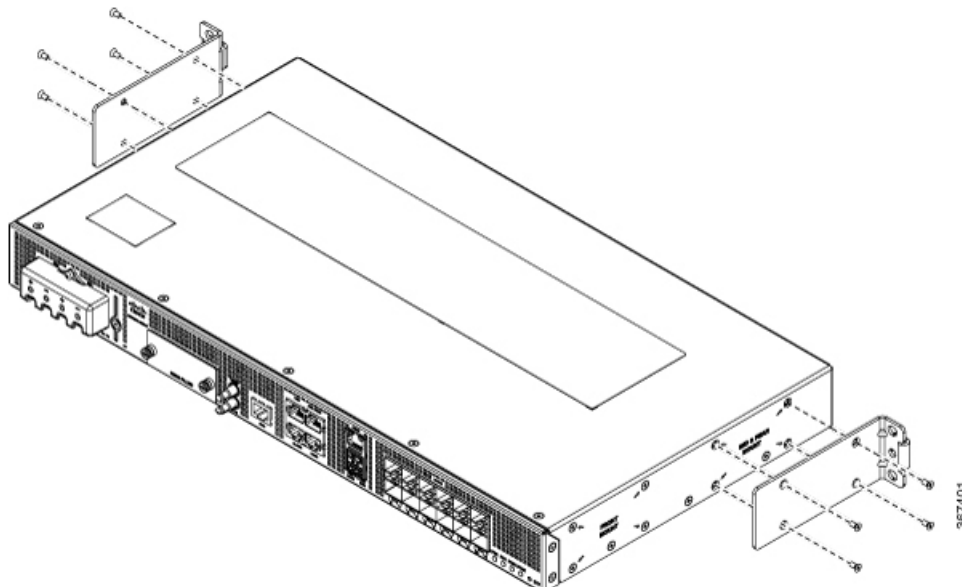
Figura 7: Instalación de los soportes de montaje en el router para un rack EIA de 19 pulgadas (posición trasera)
