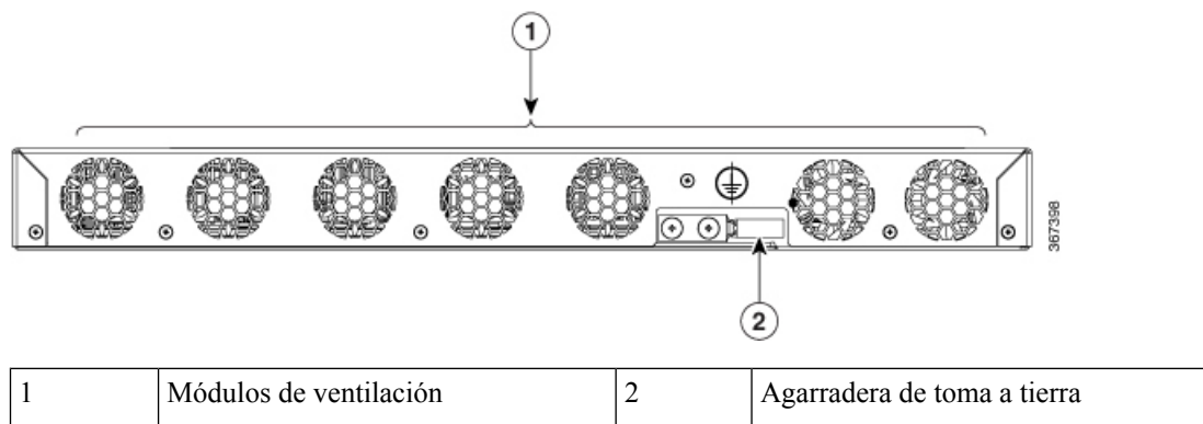
Figura 3: Vista del panel trasero del Cisco ASR-920-12SZ
