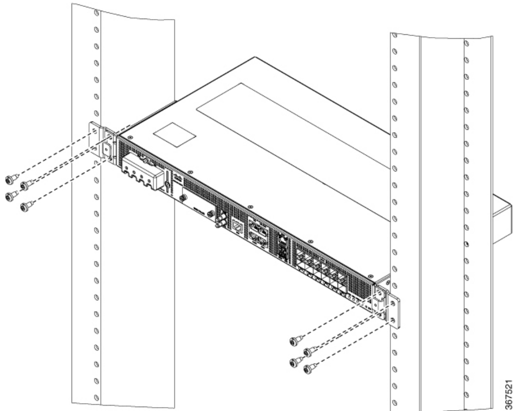
Figura 11: Configuración del dispositivo en rack de 21 pulgadas (montaje delantero)
