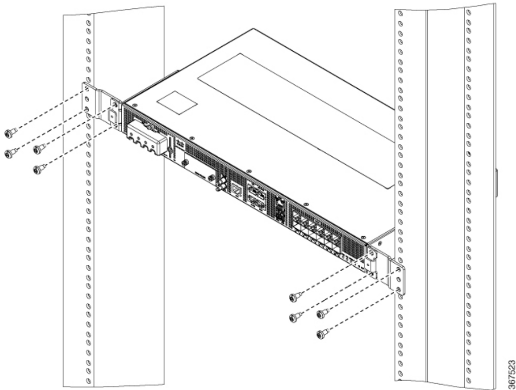
Figura 12: Configuración del dispositivo en rack de 23 pulgadas (montaje delantero)
