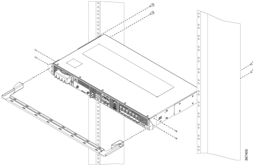
Figura 16: Dispositivo de montaje delantero con guía de cable en rack de 21 pulgadas
