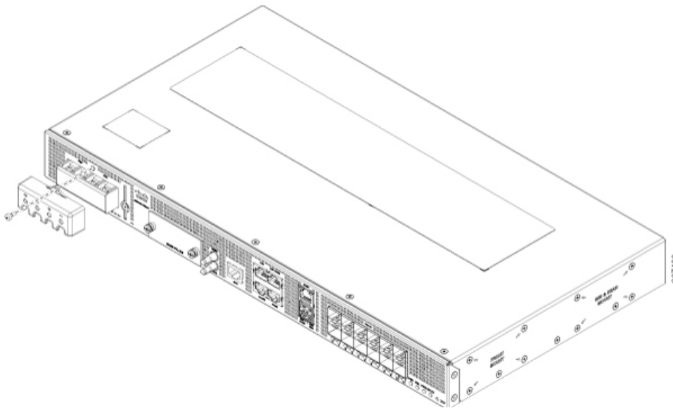
Figura 24: Protección de la fuente de alimentación de CC
