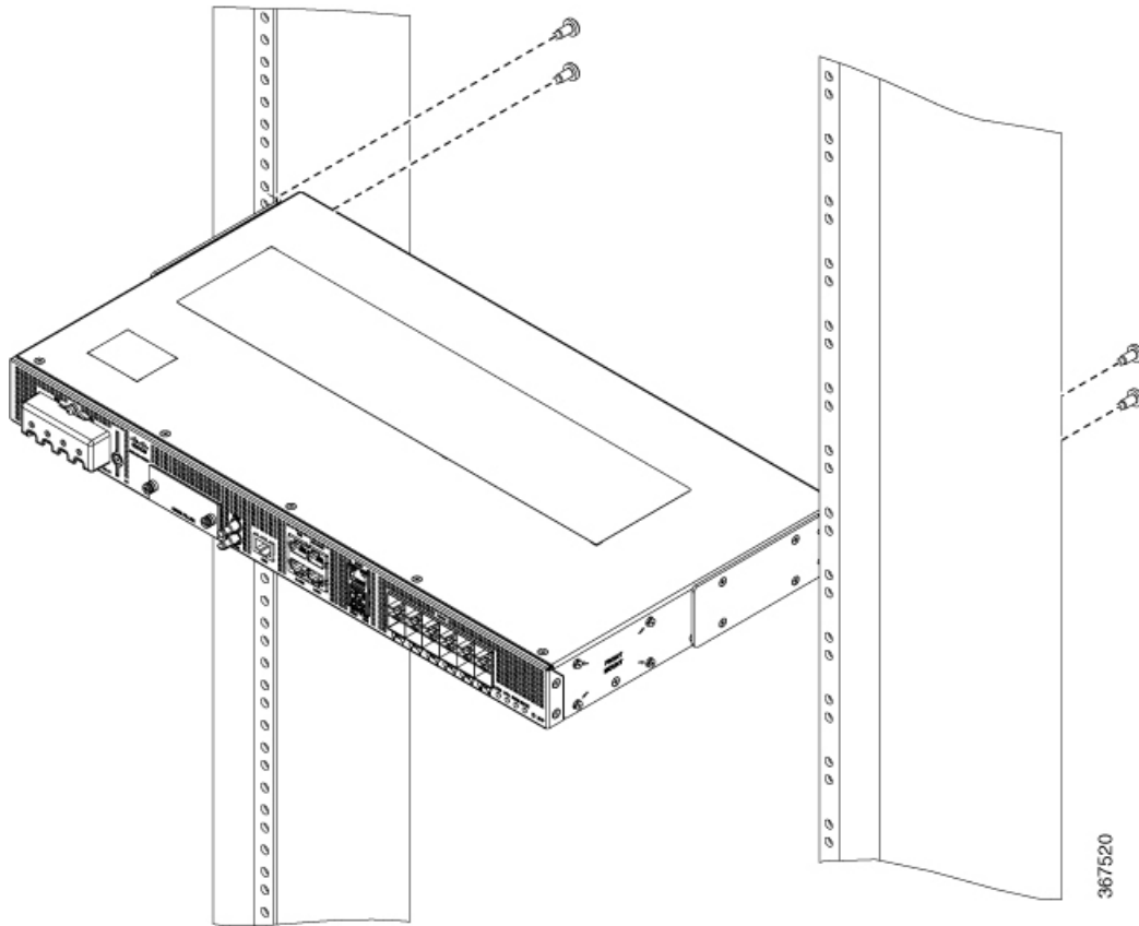
Figura 10: Configuración del dispositivo en rack de 19 pulgadas (montaje trasero)
