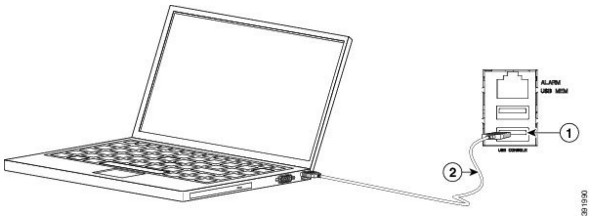
Figura 27: Conexión del cable de consola USB al router Cisco ASR 920
