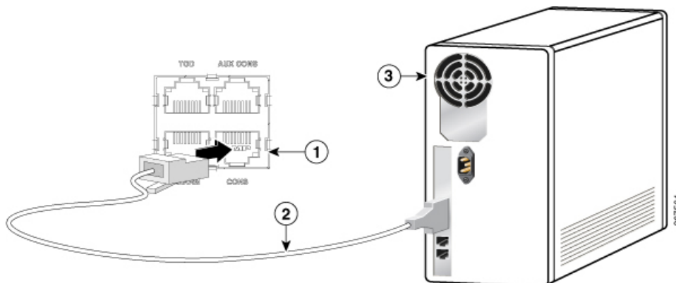
Figura 30: Conexión de un módem al router
