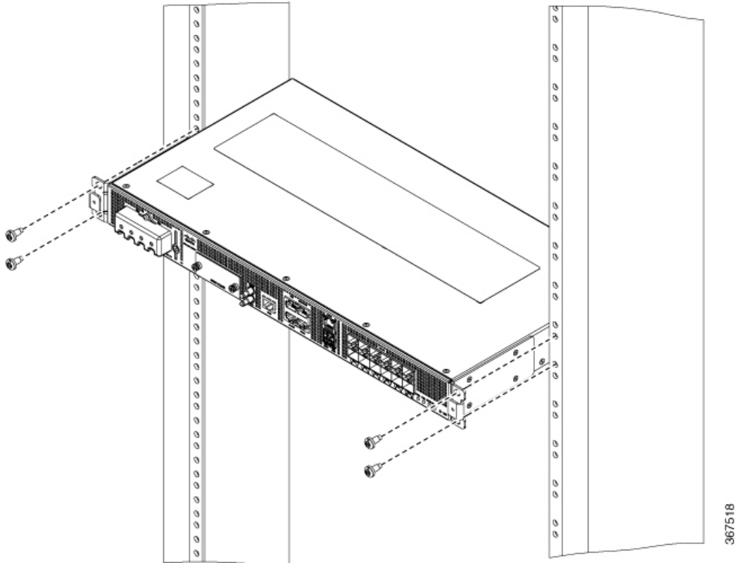
Figura 8: Configuración del dispositivo en rack de 19 pulgadas (montaje delantero)
