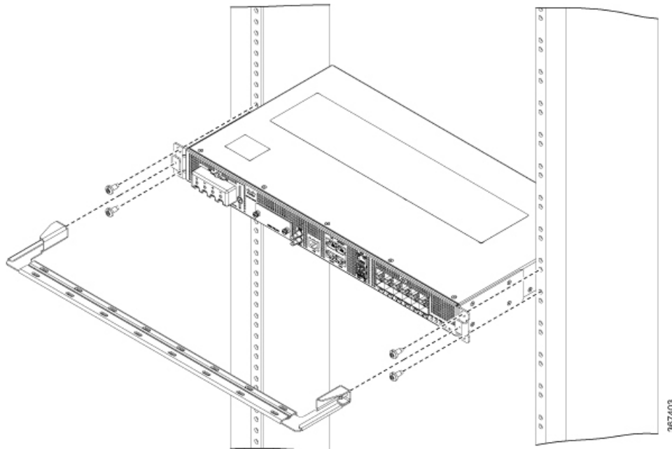
Figura 14: Dispositivo de montaje central con guía de cable en rack de 19 pulgadas
