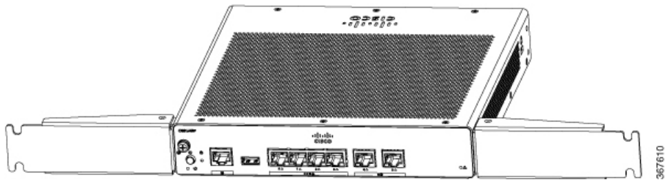
Illustration 21 : Routeur avec support fixé au panneau avant
