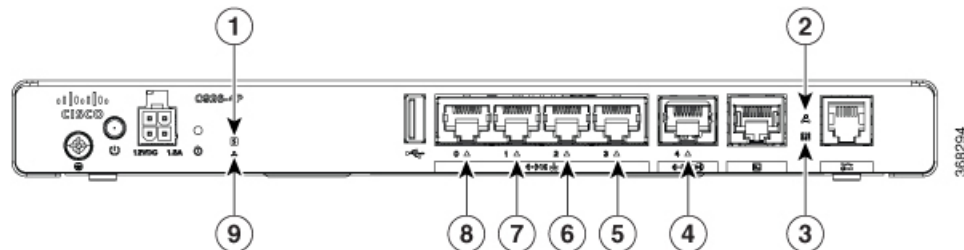
Illustration 16 : Voyants côté E/S sur les références DSL
