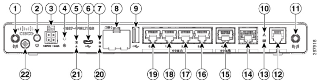
Figura 12: Cisco C927-4PMLTEGB: vista de E/S
