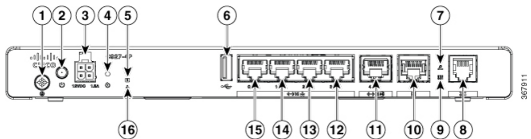
Figura 9: Cisco C927-4P: vista de E/S
