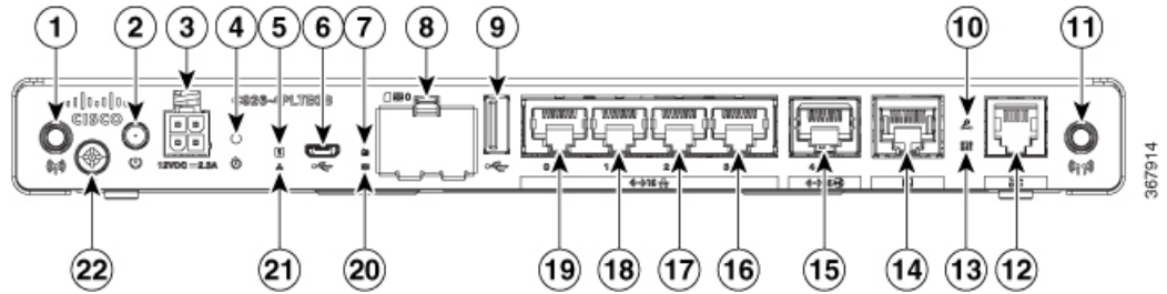
Figura 8: Cisco C926-4PLTEGB: vista de E/S
