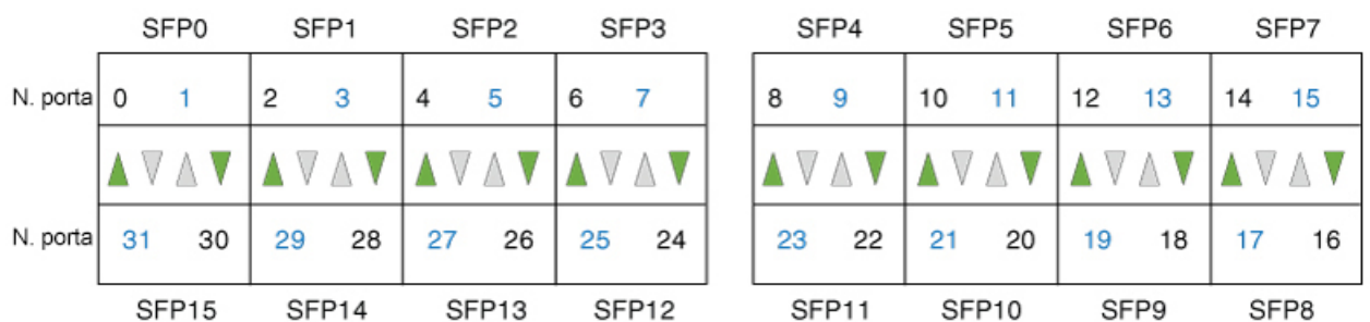
Figura 38: Porte SFP con collegamento attivo su adattatore modulare per porte Gigabit Ethernet a 32 porte con MACsec
