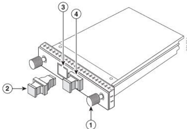
Figura 70: Ricetrasmittitore CFP
