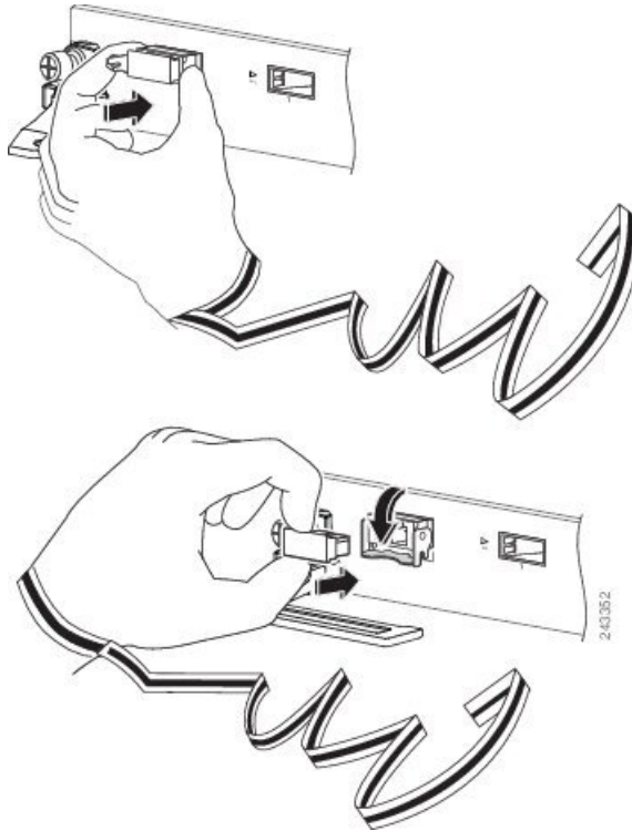
Figura 67: Installazione del modulo ricetrasmittitore XFP 10 Gigabit Ethernet
