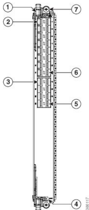
Figura 8: Scheda di linea 10 Gigabit Ethernet/Gigabit Ethernet a 24 porte
