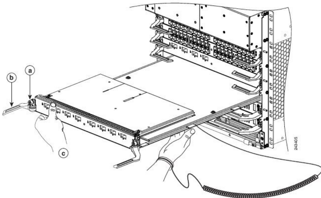
Figura 45: Rimozione di una scheda di linea (Cisco ASR 9922 Router in figura)
