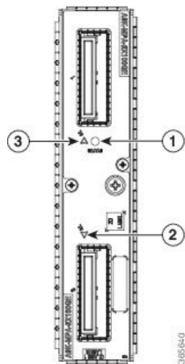
Figura 29: Adattatore modulare per porte 100 Gigabit Ethernet a 2 porte con CFP2
