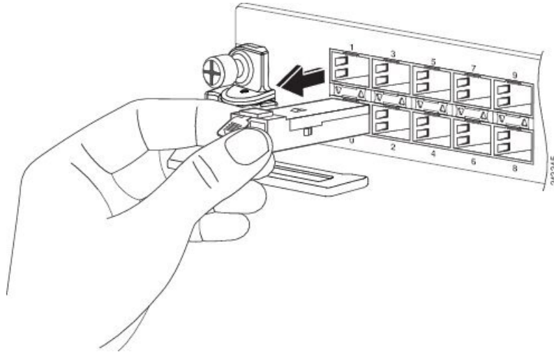
Figura 58: Rimozione di un modulo SFP con linguetta in mylar
