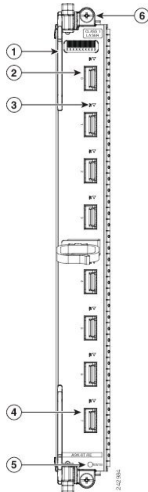
Figura 2: Scheda di linea 10 Gigabit Ethernet a 8 porte con oversubscription 2:1
