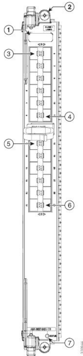
Figura 7: Scheda di linea 10 Gigabit Ethernet a 24 porte
