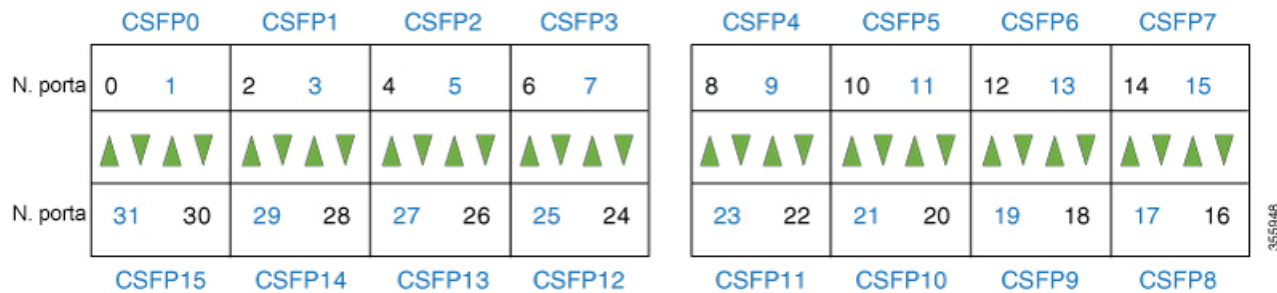
Figura 40: Porte CSFP su un adattatore modulare per porte Gigabit Ethernet a 32 porte con MACsec
