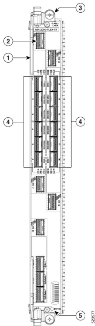
Figura 21: Scheda di linea 100 Gigabit Ethernet a 20 porte con QSFP28/QSFP-DD
