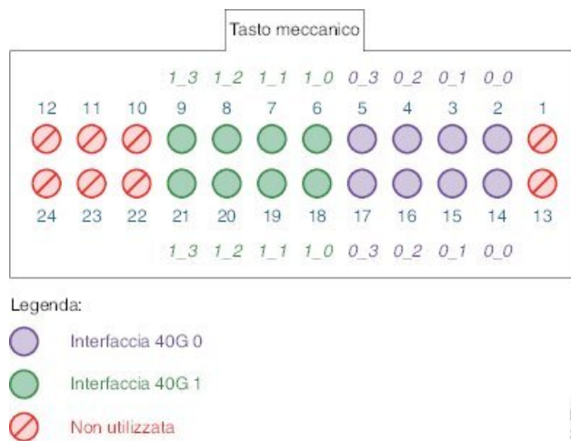
Figura 93: Pinout del connettore MPO-24 100 Gigabit (modalità 2x40)
