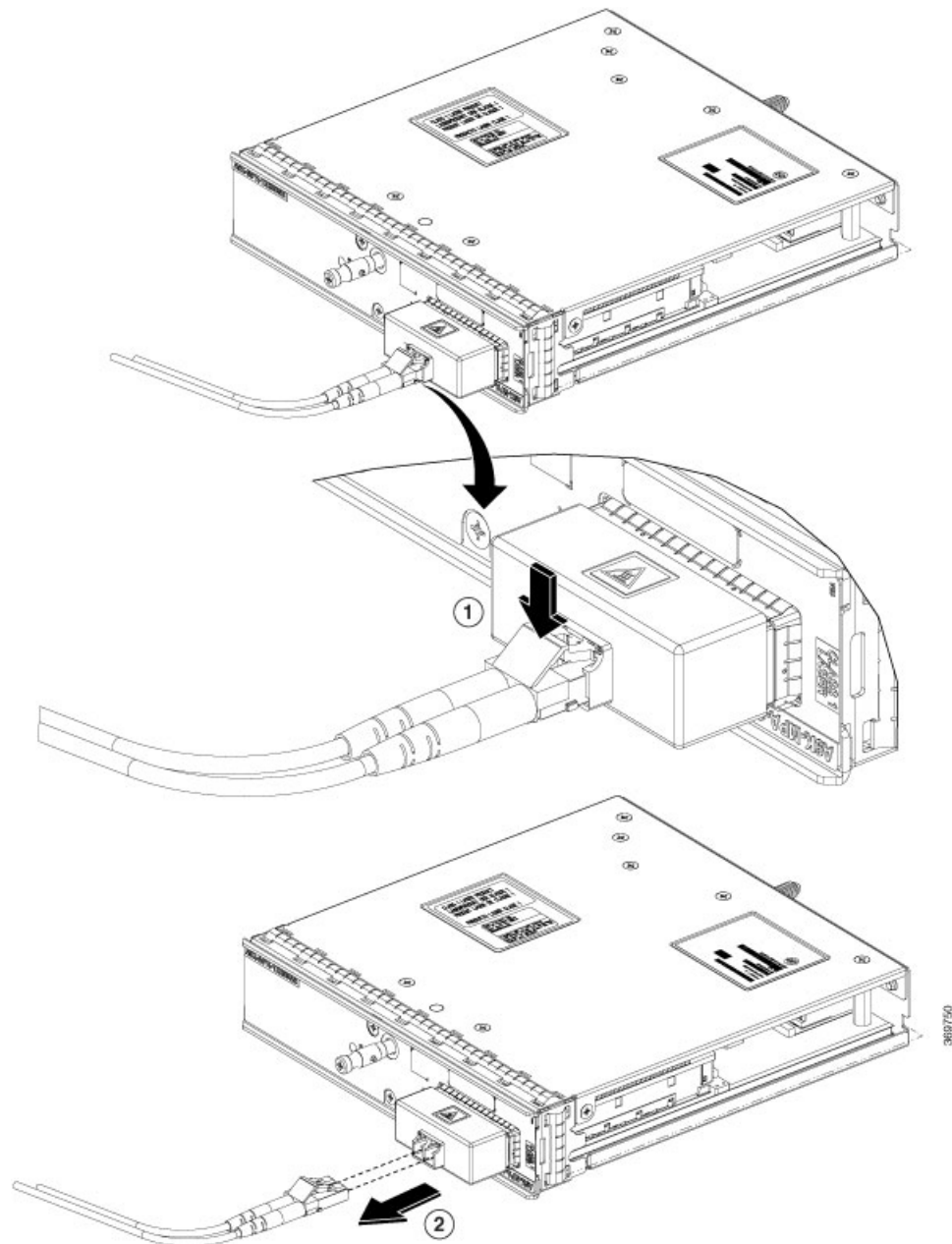
Figura 50: Rimozione dei moduli CFP2-DCO
