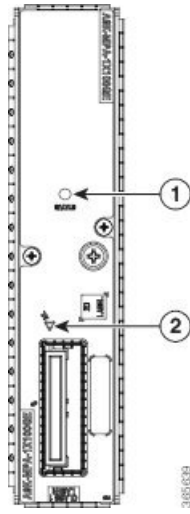
Figura 27: Adattatore modulare per porte 100 Gigabit Ethernet a 1 porta con CFP2
