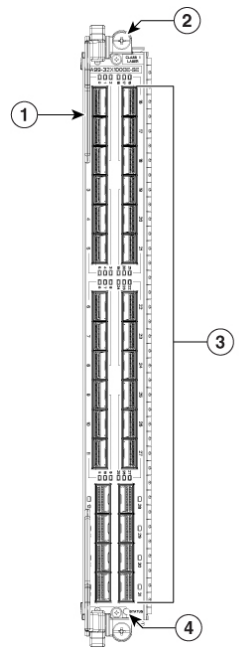
Figura 20: Scheda di linea 100 Gigabit Ethernet a 32 porte con QSFP28/QSFP+
