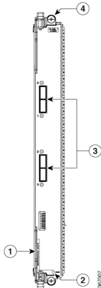
Figura 18: Scheda di linea 100 Gigabit Ethernet a 4 porte con QSFP28
