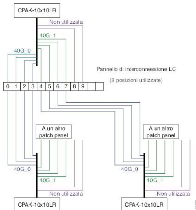
Figura 95: Cavo breakout in fibra ottica per 10x10LR CPAK-to-CPAK (modalità 2x40G facoltativa)
