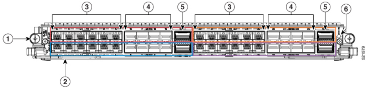
Figura 25: Scheda di linea multi-rate 400G combinata
