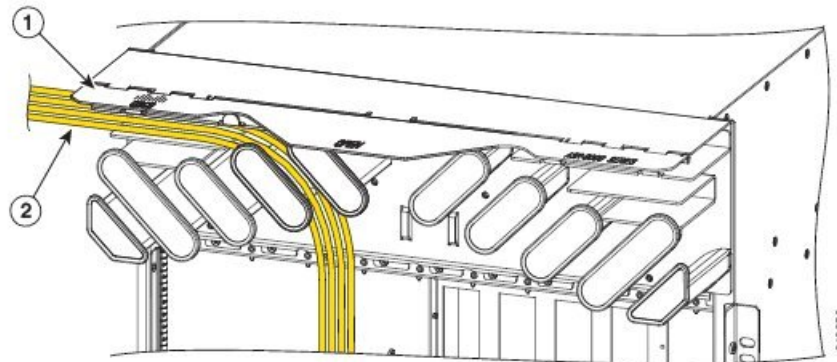
Figura 83: Esempio di cavi disposti lungo il vassoio di gestione sul router Cisco ASR 9010
