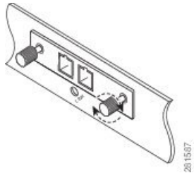
Figura 73: Fissaggio di un modulo ricetrasmittitore CFP
