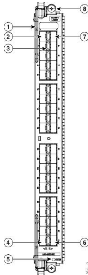
Figura 11: Scheda di linea Ethernet Gigabit a 40 porte (scheda di linea A9K-40GE-SE in figura)
