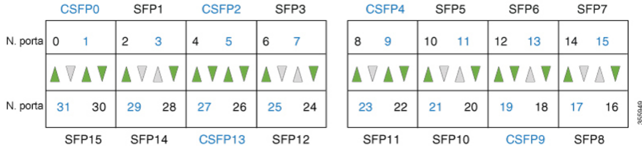
Figura 39: Porte SFP e CSFP su un adattatore modulare per porte Gigabit Ethernet a 32 porte con MACsec
