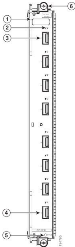
Figura 4: Scheda di linea 10 Gigabit Ethernet a 8 porte da 80 Gbps
