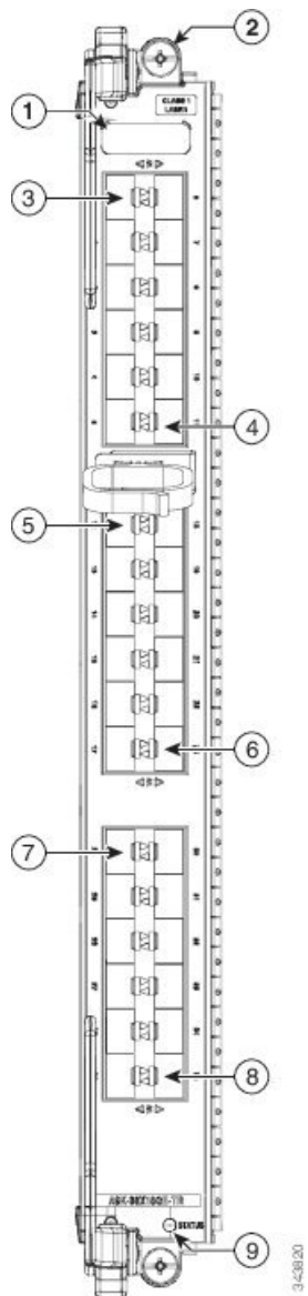
Figura 9: Pannello anteriore della scheda di linea 10 Gigabit Ethernet a 36 porte
