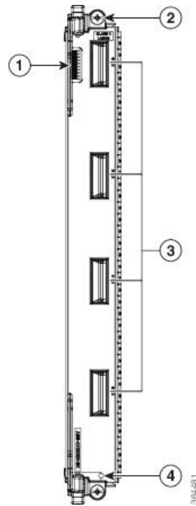
Figura 14: Scheda di linea 100 Gigabit Ethernet a 4 porte
