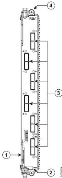
Figura 19: Scheda di linea 100 Gigabit Ethernet a 12 porte con QSFP28
