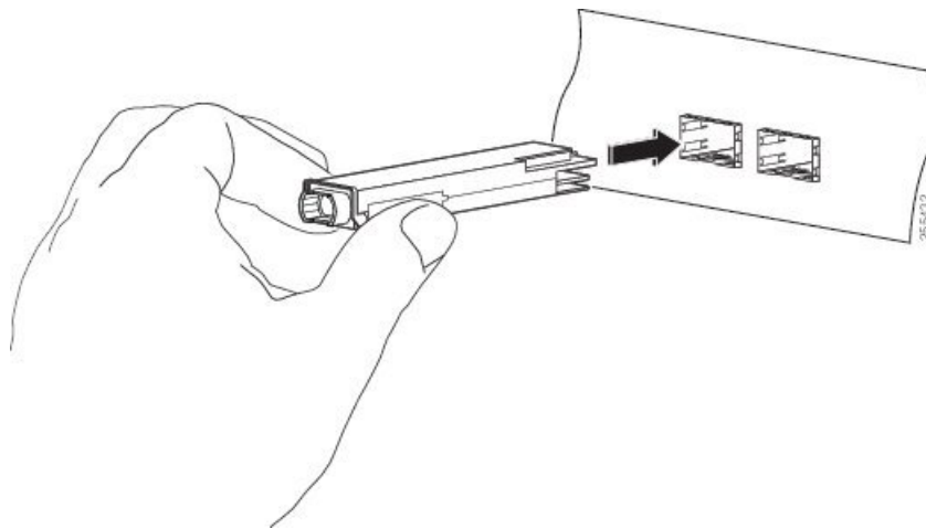
Figura 77: Installazione del modulo ricetrasmittitore QSFP+ 40 Gigabit o QSFP28 100 Gigabit (modulo ricetrasmittitore ottico con levetta di chiusura in figura)
