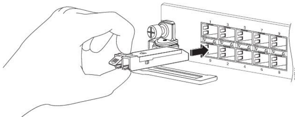
Figura 57: Installazione di un modulo SFP con linguetta in mylar
