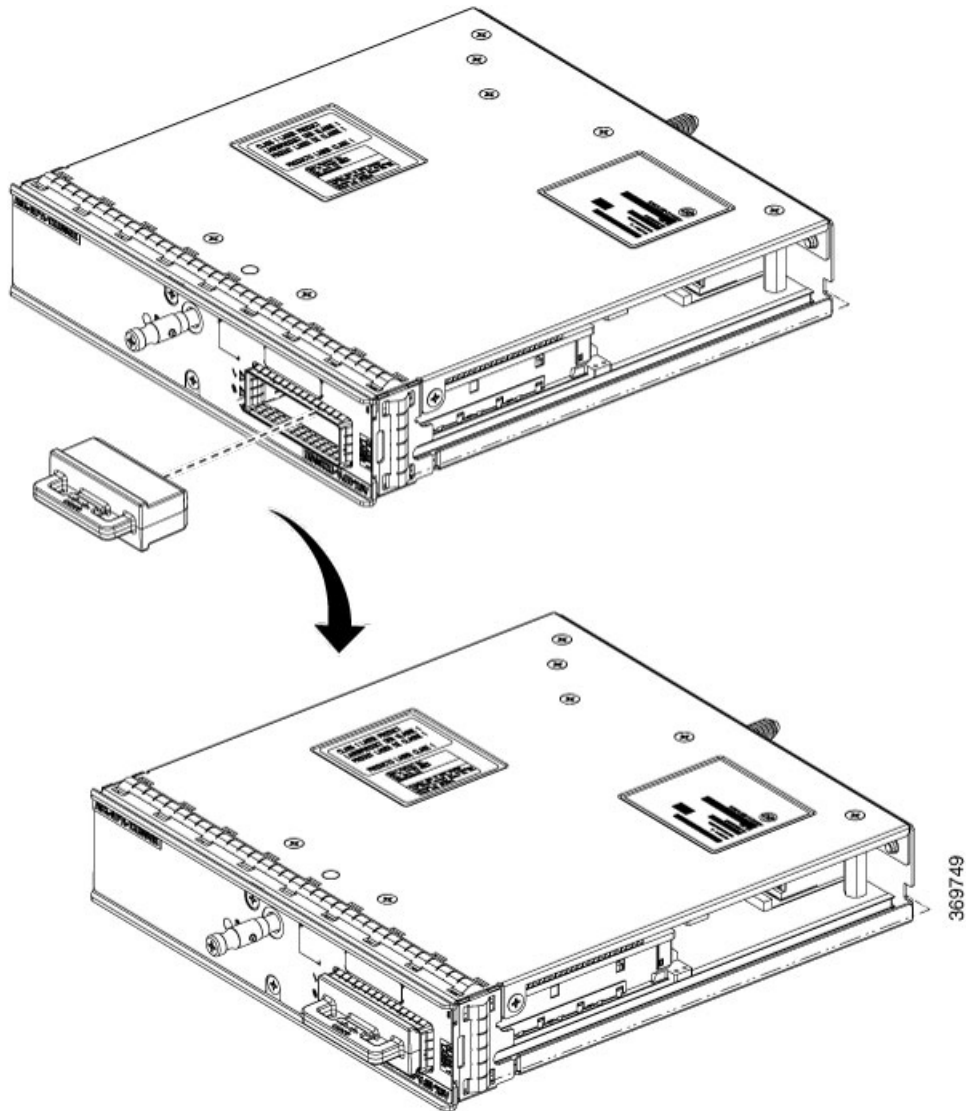
Figura 51: Coprire la porta con il tappo antipolvere CFP2
