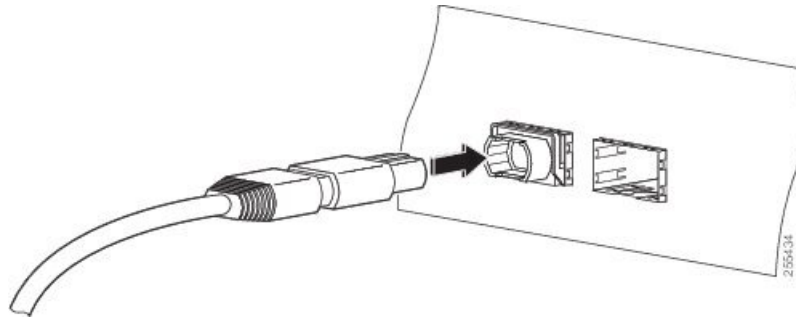
Figura 79: Cablaggio di un modulo ricetrasmittitore QSFP+ o QSFP28 40 Gigabit
