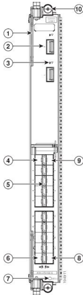
Figura 1: Scheda di linea combinata 10 Gigabit a 2 porte + GE a 20 porte
