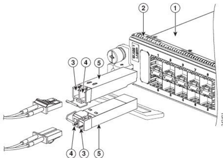
Figura 87: Modulo SFP e cavo in fibra ottica
