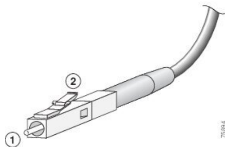
Figura 88: Connettore per cavi LC simplex
