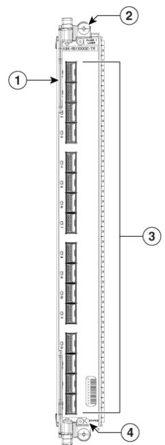
Figura 16: Scheda di linea 100 Gigabit Ethernet a 16 porte con QSFP28/QSFP+
