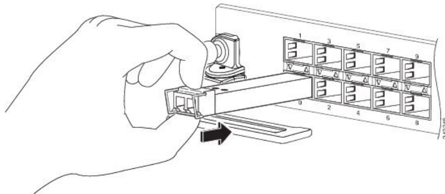
Figura 54: Installazione di un modulo SFP con levetta di chiusura in una porta
