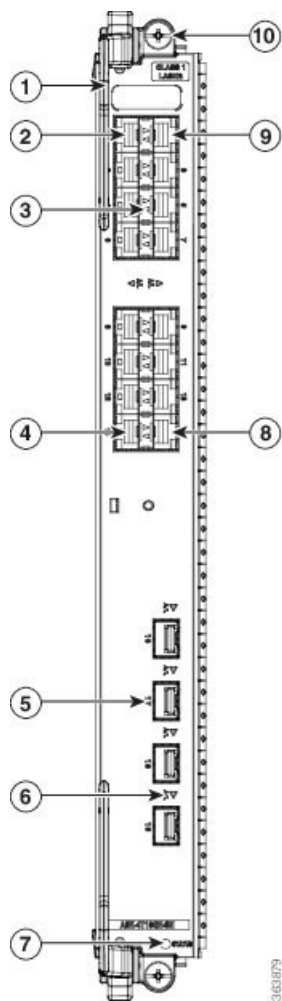
Figura 5: Scheda di linea combinata 10 Gigabit a 4 porte + GE a 16 porte
