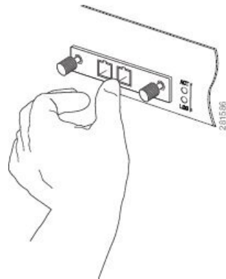
Figura 72: Inserimento del modulo ricetrasmittitore CFP nel socket
