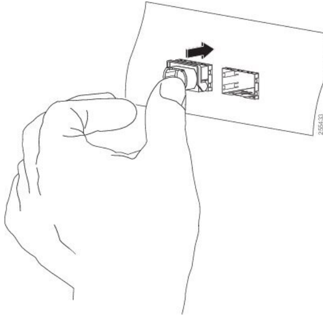
Figura 78: Inserimento nel connettore del modulo ricetrasmittitore QSFP+ 40 Gigabit o QSFP28 100 Gigabit (ricetrasmittitore ottico con levetta di chiusura in figura)
