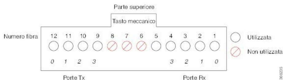
Figura 91: Pinout del connettore MPO-12 100 Gigabit
