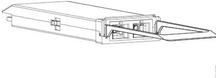
Figura 81: Esempio di modulo ricetrasmittitore CPAK 100 Gigabit Ethernet
