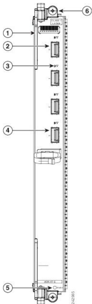
Figura 3: Scheda di linea 10 Gigabit Ethernet a 4 porte
