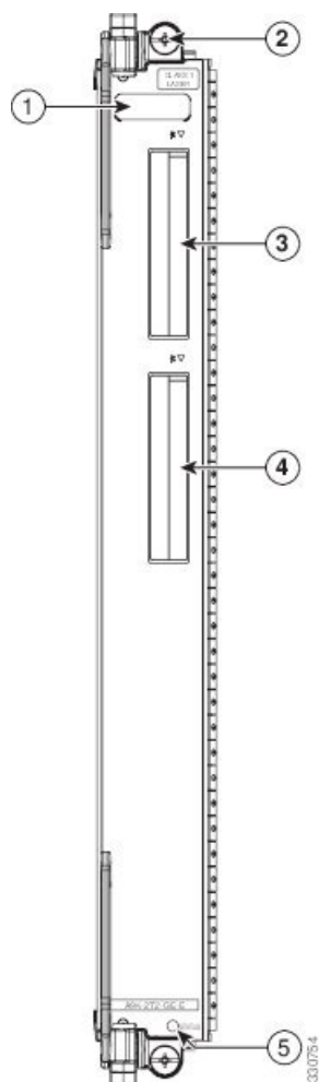
Figura 13: Scheda di linea 100 Gigabit Ethernet a 2 porte
