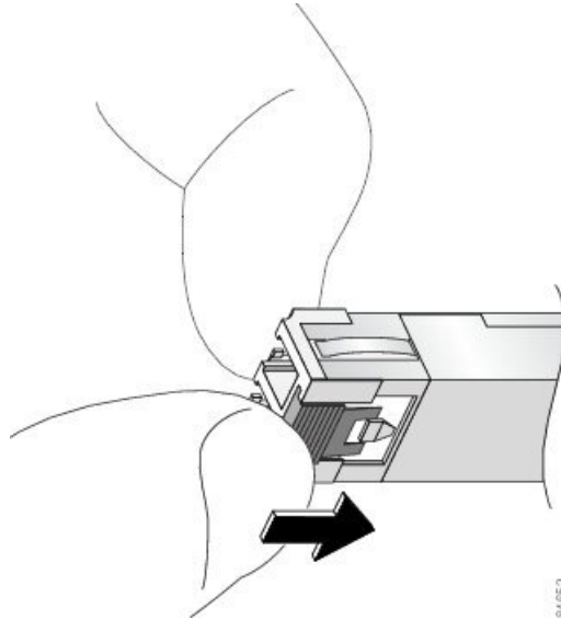
Figura 64: Disinsediamento con la linguetta scorrevole
