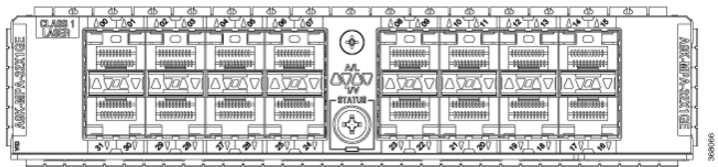
Figura 41: MPA Gigabit Ethernet a 32 porte con MACsec
