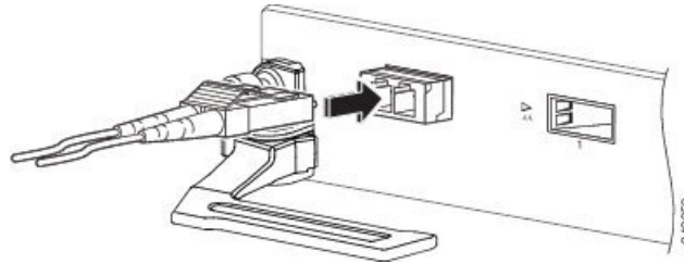
Figura 69: Cablaggio di un modulo ricetrasmittitore XFP 10 Gigabit Ethernet
