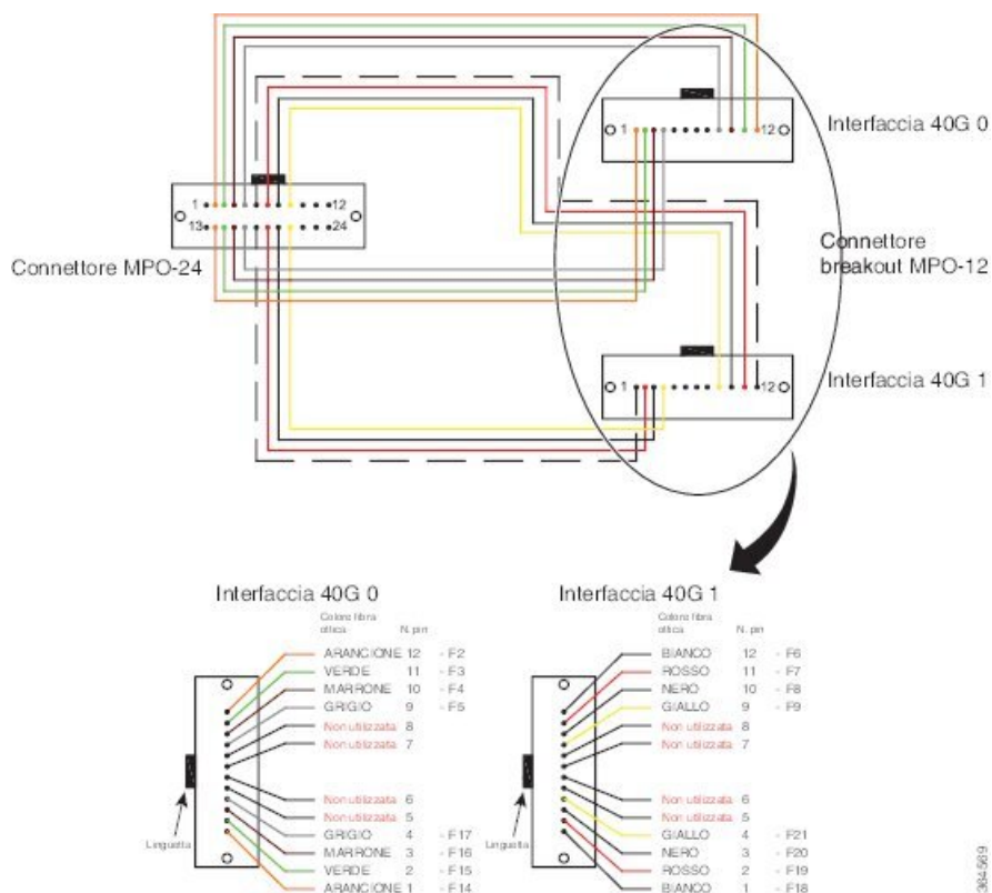
Figura 94: Cavo breakout 2x40GE per modulo ottico CPAK-100G-SR10
