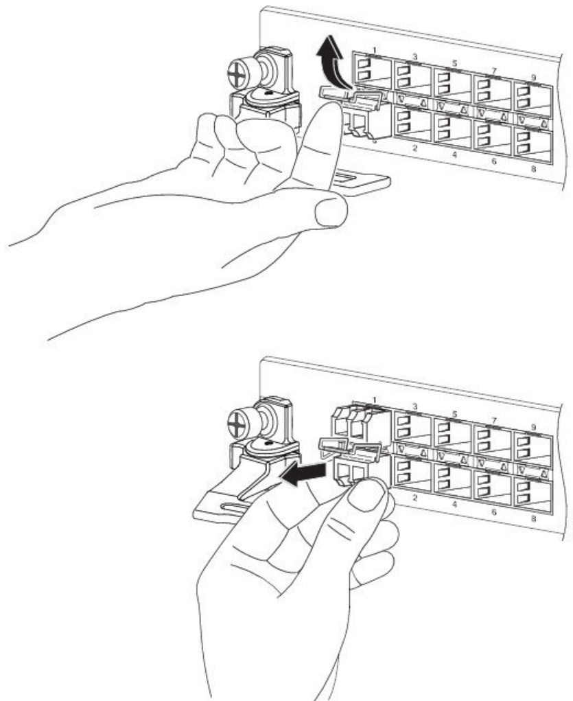
Figura 55: Rimozione di un modulo SFP o SFP+ con levetta di chiusura
