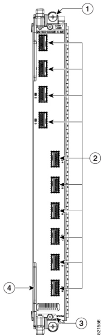
Figura 23: Scheda di linea 400 Gigabit Ethernet a 10 porte con QSFP-DD
