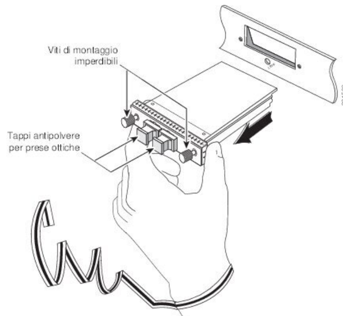
Figura 75: Rimozione di un modulo ricetrasmittitore CFP
