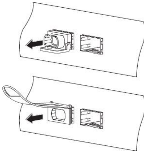
Figura 80: Rimozione del modulo ricetrasmittitore QSFP+ 40 Gigabit o QSFP28 100 Gigabit
