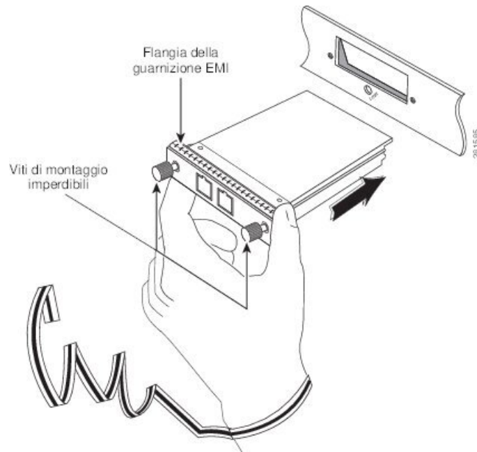
Figura 71: Installazione di un modulo ricetrasmittitore CFP
