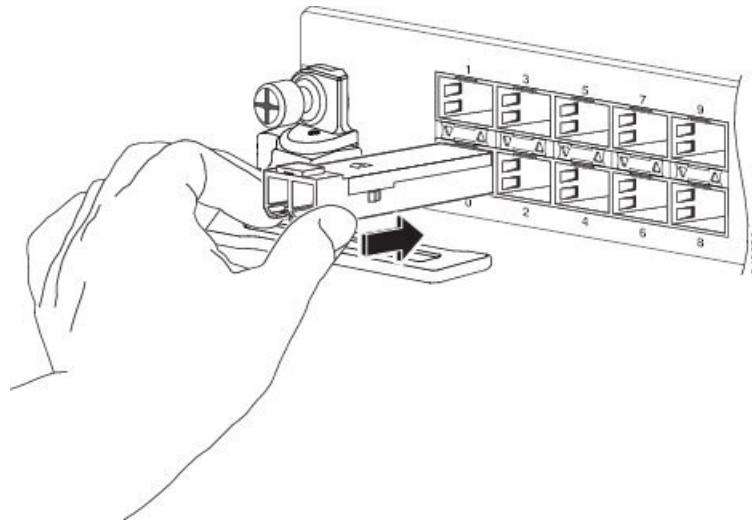
Figura 63: Installazione di un modulo SFP o SFP+ con linguetta scorrevole
