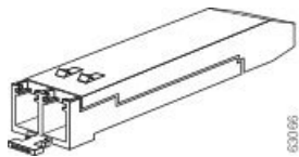
Figura 59: Modulo SFP o SFP+ con pulsante
