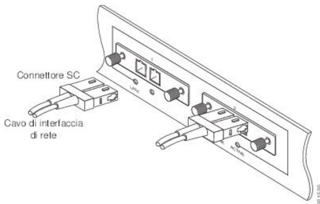
Figura 74: Cablaggio di un modulo ricetrasmittitore ottico CFP con connettori SC
