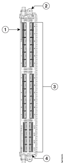
Figura 17: Scheda di linea 100 Gigabit Ethernet a 32 porte con QSFP28/QSFP+
