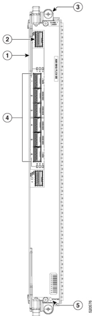
Figura 22: Scheda di linea 100 Gigabit Ethernet a 8 porte con QSFP28/QSFP-DD
