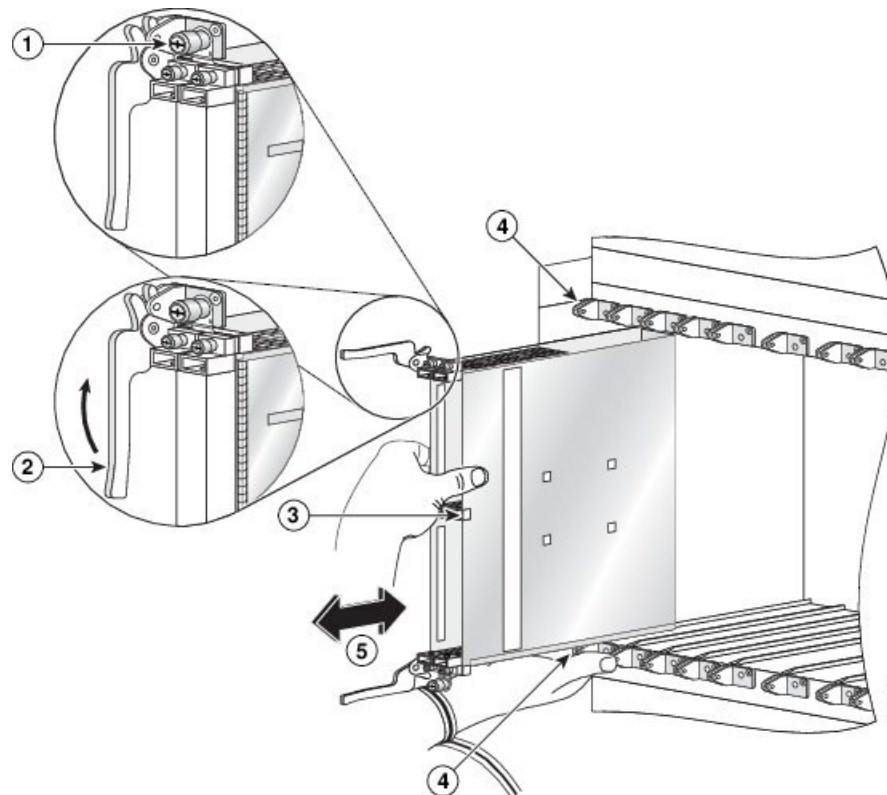
Figura 47: Rimozione e installazione di una scheda di linea modulare
