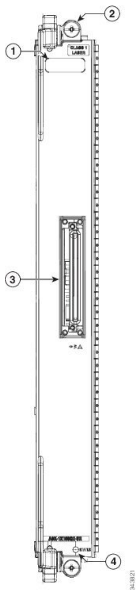
Figura 12: Pannello anteriore della scheda di linea 100 Gigabit Ethernet a 1 porta
