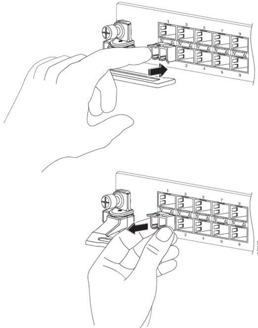
Figura 61: Rimozione di un modulo SFP o SFP+ con pulsante da una porta
