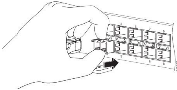
Figura 60: Installazione di un modulo SFP o SFP+ con pulsante
