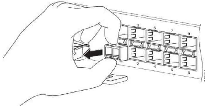
Figura 65: Rimozione di un modulo SFP o SFP+ con linguetta scorrevole
