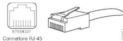
Figura 90: Connettore per cavo RJ-45
