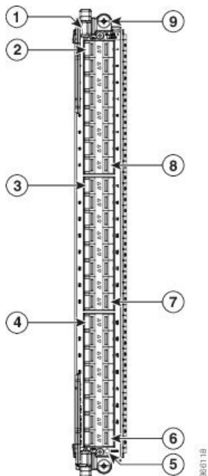
Figura 10: Scheda di linea 10 Gigabit Ethernet/Gigabit Ethernet a 48 porte
