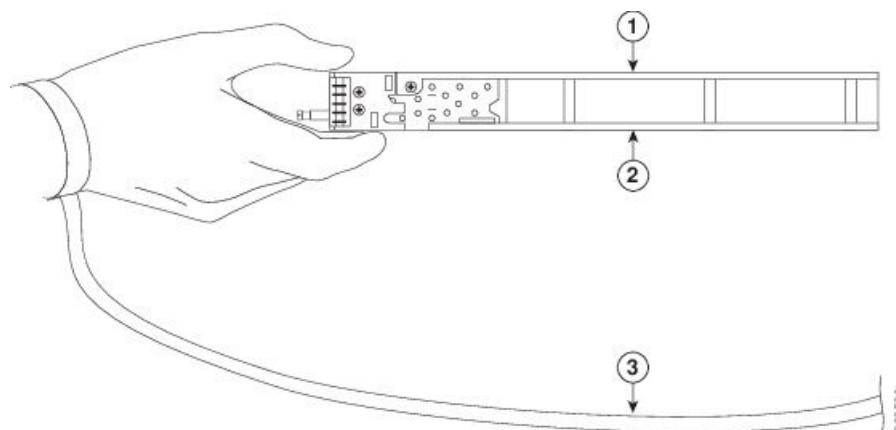
Figura 49: Come maneggiare un adattatore modulare per porte
