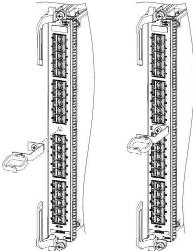
Figura 86: Installazione e rimozione della staffa di gestione dei cavi
