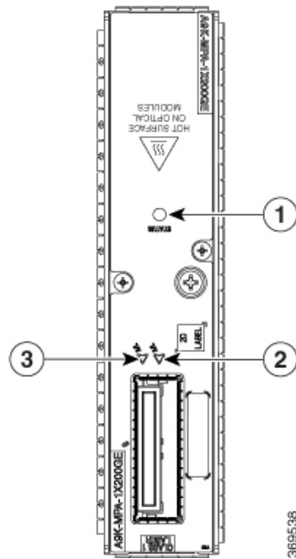
Figura 28: Adattatore modulare per porte 200 Gigabit Ethernet a 1 porta con CFP2-DCO
