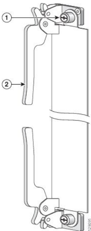
Figura 48: Levette di espulsione e viti imperdibili
