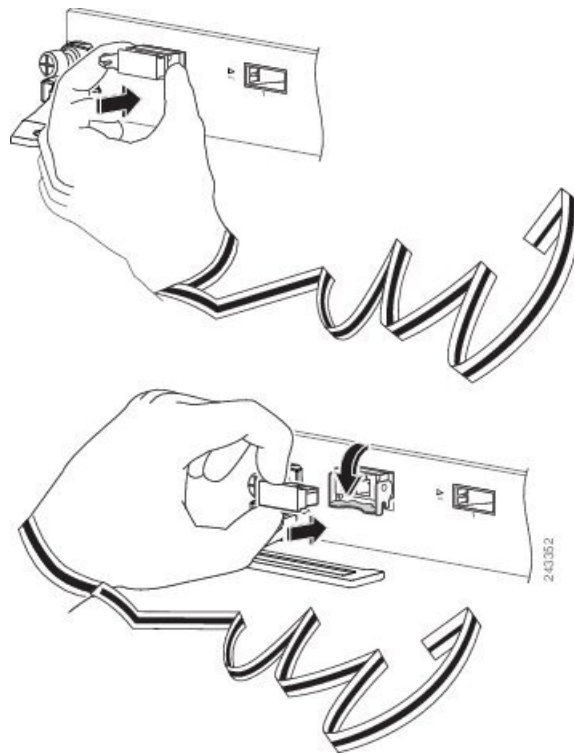
Figura 66: Modulo ricetrasmittitore XFP 10 Gigabit Ethernet
