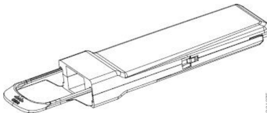
Figura 82: Modulo adattatore CPAK
